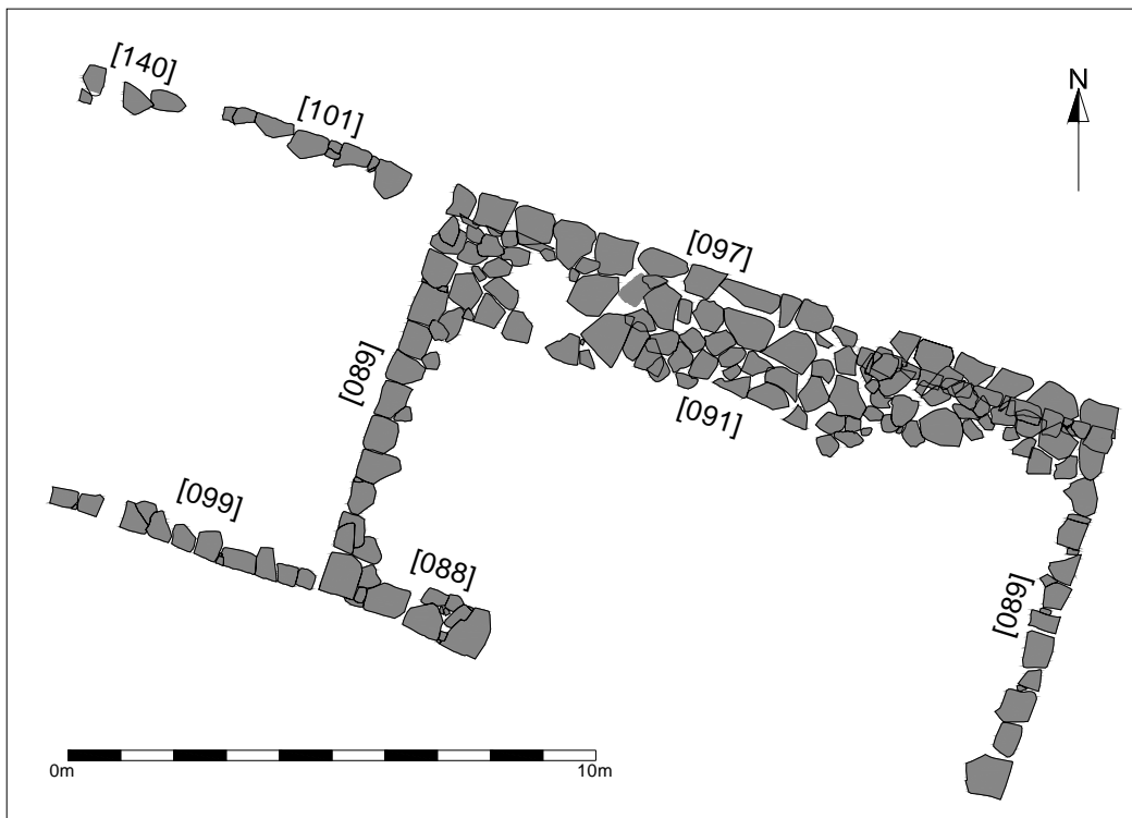
Mynd 13: Yfirlitsteikning sem sýnir sökkla hússins sem stóð við Austurstræti 22 (einingar [088],[089],[097]) ásamt leifum grjóthlaðins garðs (einingar [099], [101], [140]) og yngri grjótlögn (eining [091]).
