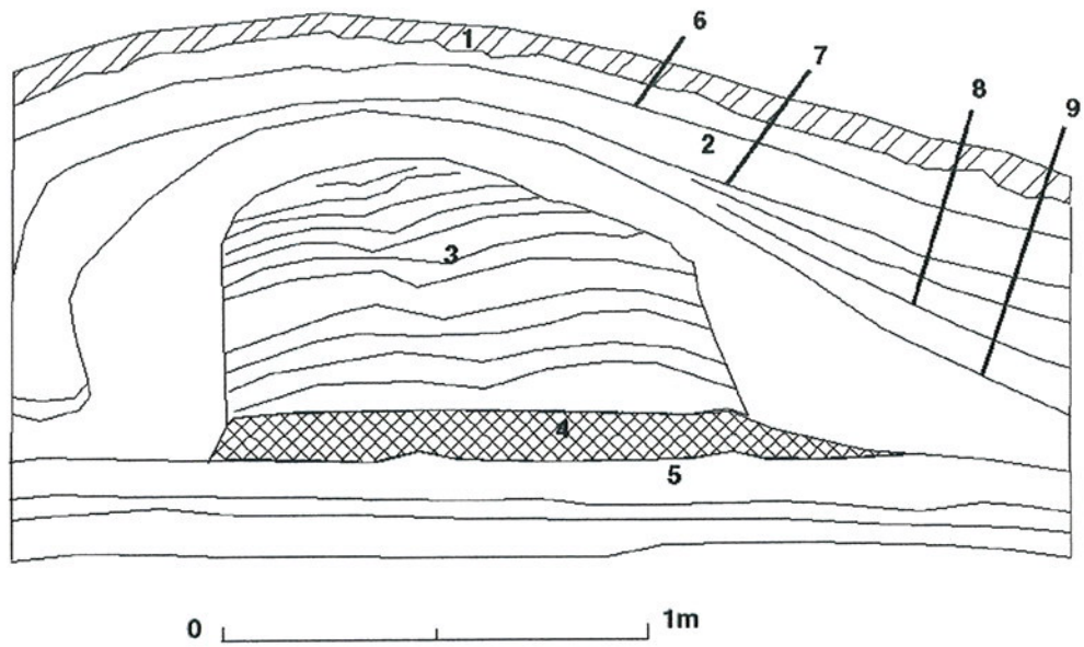
Teikning 5. Skurður 5. Austursnið.
