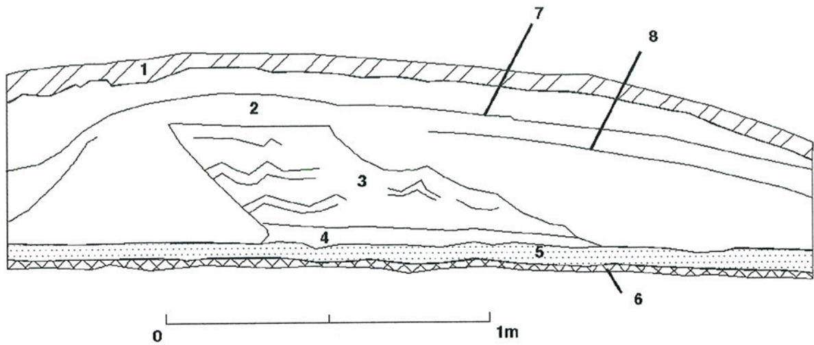
Teikning 4. Skurður 4. Austursnið.
