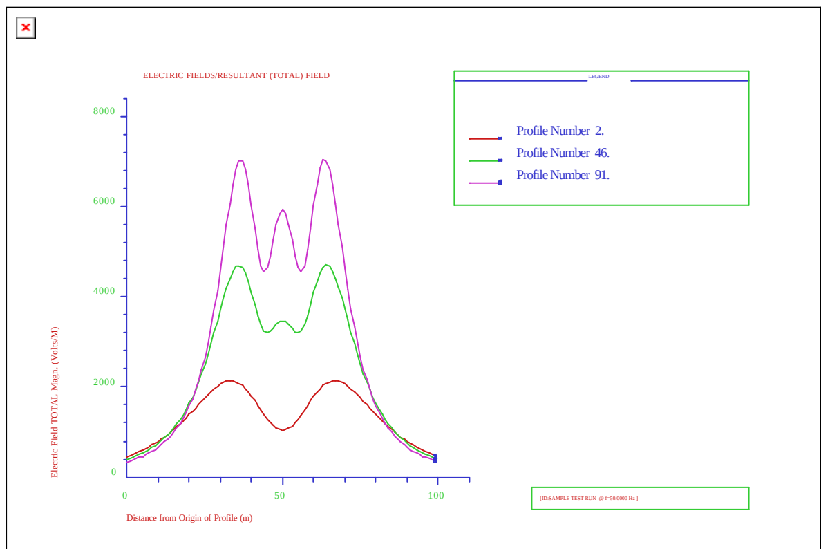
Mynd 3.2 Rafsvið í þremur sniðum undir stakstæðri Sultartangalínu 3, við mastur (neðsti ferill), í fjórðungspunkti (ferill í miðju) og á miðju hafi (efsti ferill).
