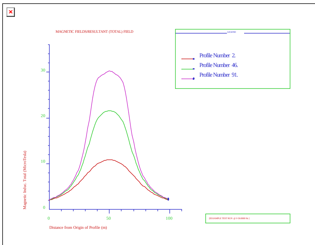
Mynd 3.4 Segulsvið í þremur sniðum undir stakstæðri Sultartangalínu 3, við mastur (neðsti ferill), í fjórðungspunkti (ferill í miðju) og á miðju hafi (efsti ferill).
