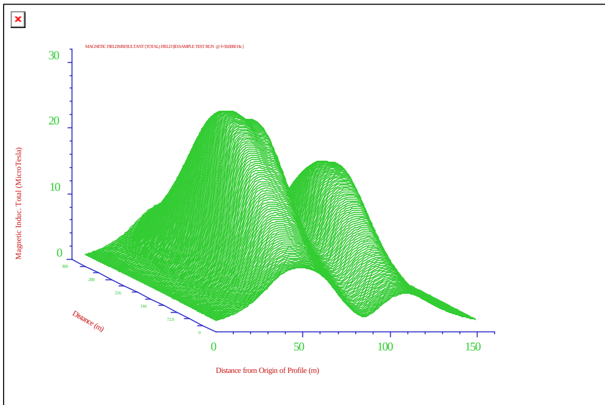
Mynd 3.7 Þrívíddarmynd af segulsviði undir samsíða Sultartangalínum 1 og 3 fyrir 360 m hafleigd. 775 MVA flutningur eftir SU3 og 300 MVA eftir SU1.
