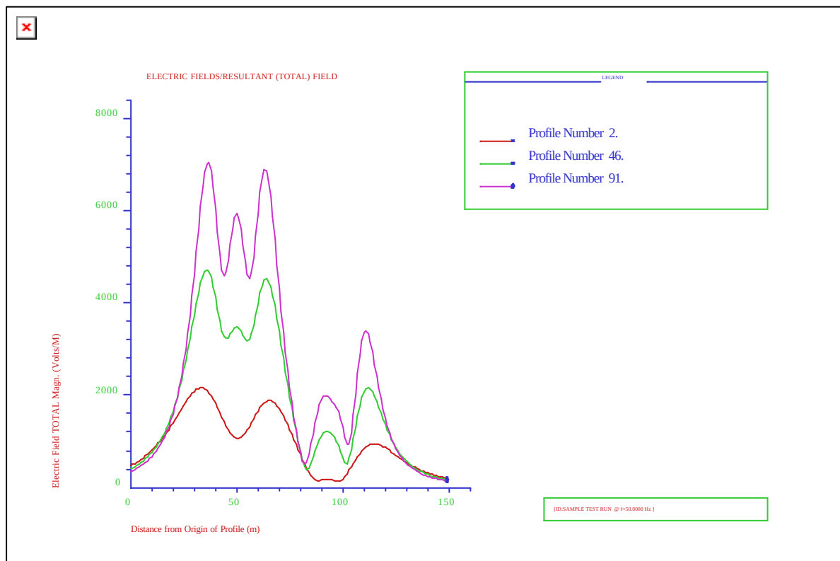
Mynd 3.6 Rafsvið í þremur sniðum undir samsíða Sultartangalínnum 1 og 3, við mastur (neðsti ferill), í fjórðungspunkti (ferill í miðju) og á miðju hafi (efsti ferill).
