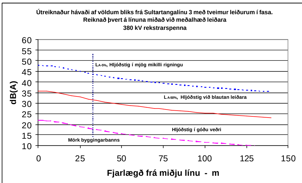
Mynd 2.1 Útreiknaður hávaði af völdum blíks frá stakstæðri Sultartangalínu 3.
