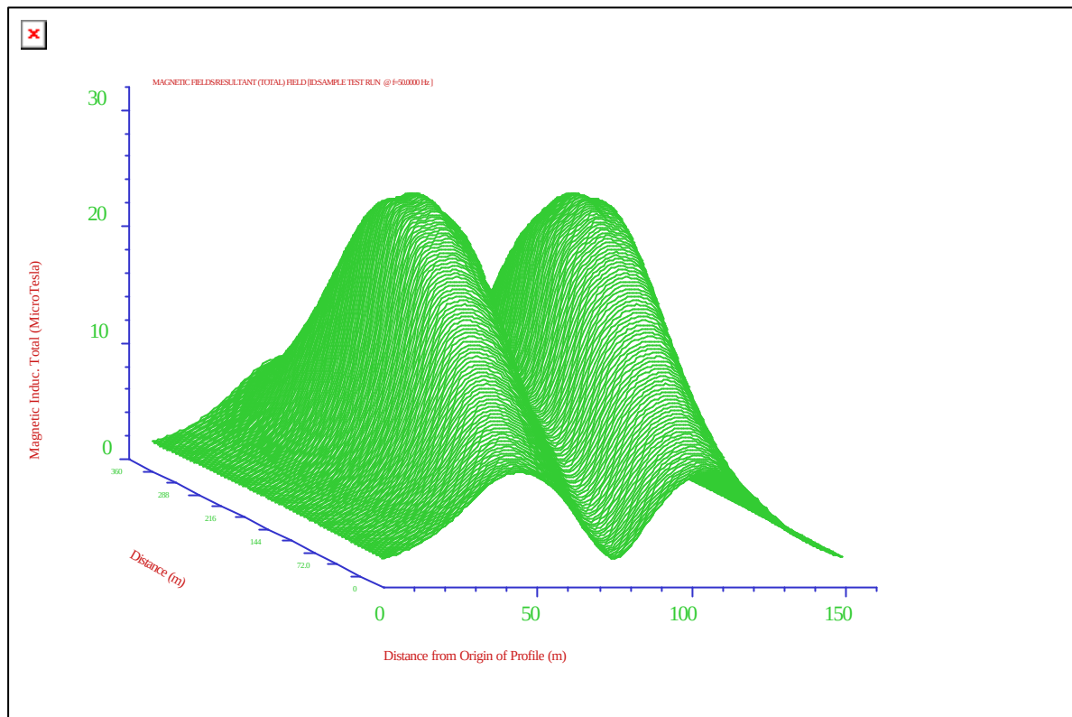
Mynd 3.11 Þrívíddarmynd af segulsviði undir samsíða Sultartangalínu 3 og 420 kV Brennimelslínu 1 fyrir 360 m haflengd. 775 MVA flutningur eftir báðum línun.
