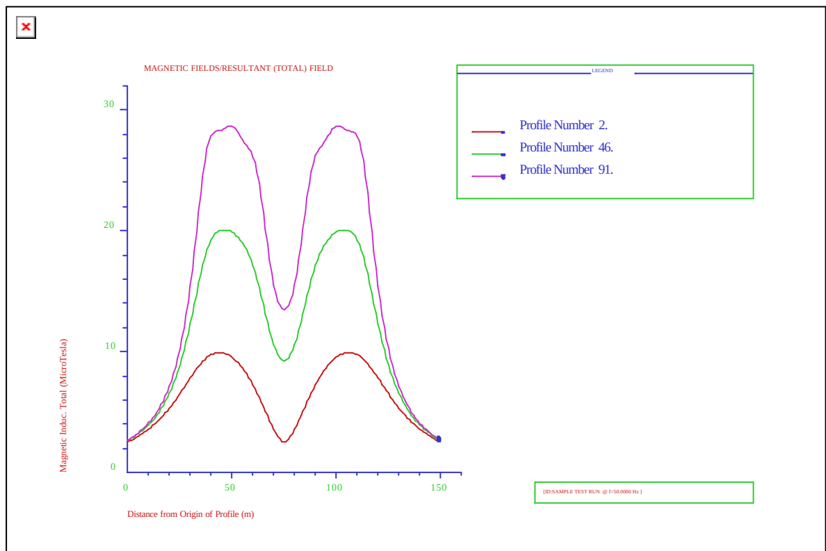
Mynd 3.12 Segulsvið í þremur sniðum undir samsíða Sultartangalínu 3 og 420 kV Brennimelslínu 1, við mastur (neðsti ferill), í fjórðungspunkti (ferill í miðju) og á miðju hafi (efsti ferill).
