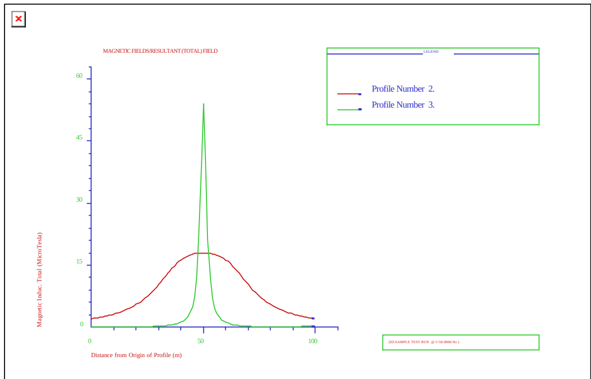
Mynd 3.13 Segulsvið Sultartangalínu 3 við áætlaða meðalhæð leiðara borið saman við segulsvið frá streng við yfirborð jarðar. Þröngi ferillinn sýnir segulsvið strengs.
