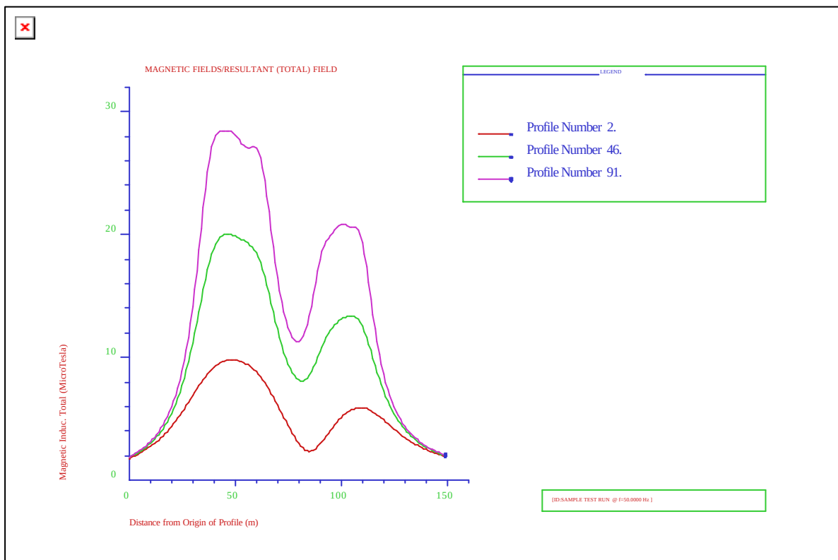
Mynd 3.8 Segulsvið í þremur sniðum undir samsíða Sultartangalínum 1 og 3, við mastur (neðsti ferill), í fjórðungspunkti (ferill í miðju) og á miðju hafi (efsti ferill).
