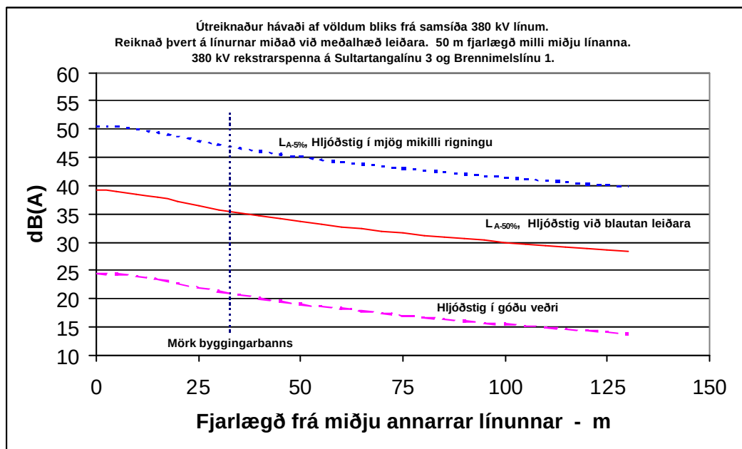
Mynd 2.3 Útreiknaður hávaði af völdum blikis frá Sultartangalínu 3 og Brennimelslínu 1 þar sem þær liggja samsíða.
