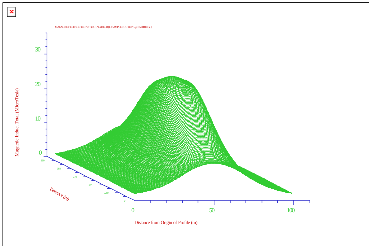
Mynd 3.3 Þrívíddarmynd af segulsviði undir stakstæðri Sultartangalínu 3 fyrir 360 m haf lengd. 775 MVA flutningur eftir línunni.
