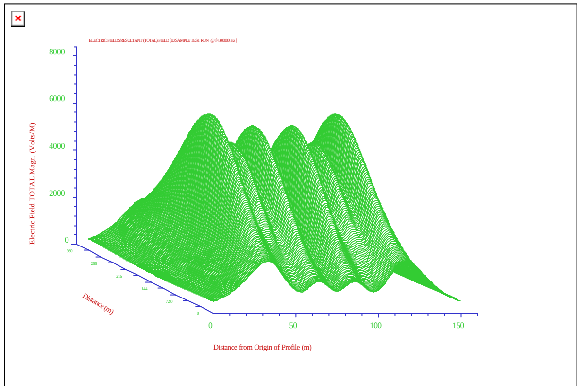
Mynd 3.9 Þrívíddarmynd af rafsviði undir samsíða Sultartangalínu 3 og 420 kV Brennimelslínu 1 fyrir 360 m haflengd. 380 kV rekstrarspenna á báðum línun.
