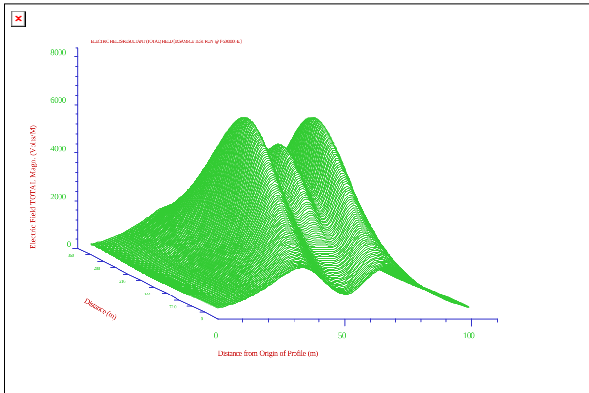
Mynd 3.1 Þrívíddarmynd af rafsviði undir stakstæðri Sultartangalínu 3 fyrir 360 m haflengd. 380 kV rekstrarspenna.
