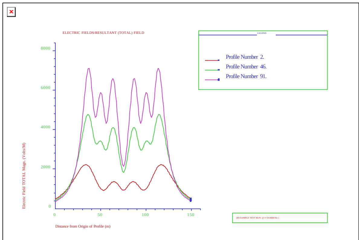
Mynd 3.10 Rafsvið í þremur sniðum undir samsíða samsíða Sultartangalínu 3 og 420 kV Brennimelslínu 1, við mastur (neðsti ferill), í fjórðungspunkti (ferill í miðju) og á miðju hafi (efsti ferill).
