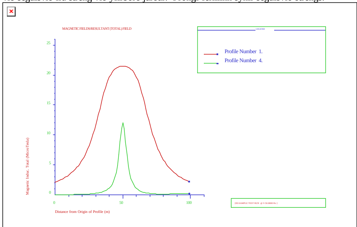
Mynd 3.14 Segulsvið Sultartangalínu 3 við áætlaða meðalhæð leiðara borið saman við segulsvið frá streng í 1,8 m hæð yfir jörðu. Þröngi ferillinn sýnir segulsvið strengs.
