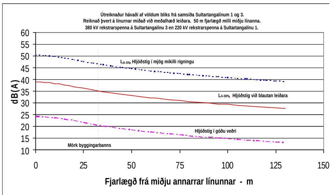
Mynd 2.2 Útreiknaður hávaði af völdum blikis frá Sultartangalínunum 1 og 3 þar sem þær liggja samsíða. Miðað er við fjarlægð frá miðju Sultartangalínu 3 þar sem reiknað hljóðstig er hærra þeim megin.
