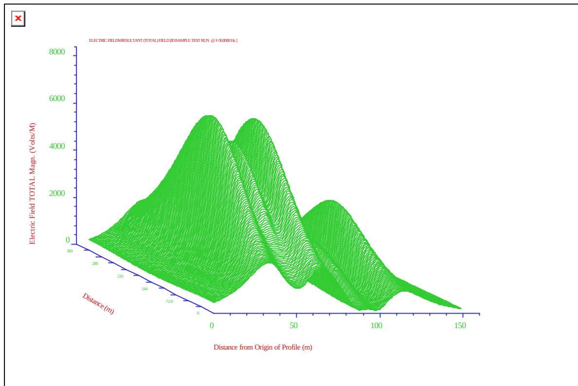
Mynd 3.5 Þrívíddarmynd af rafsviði undir samsíða Sultartangalínnum 1 og 3 fyrir 360 m haflengd. 380 kV rekstrarspenna á SU3 og 220 kV á SU1.
