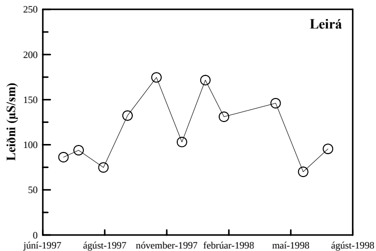
Mynd 26: Leiðni vatns í Leirá með tíma.
