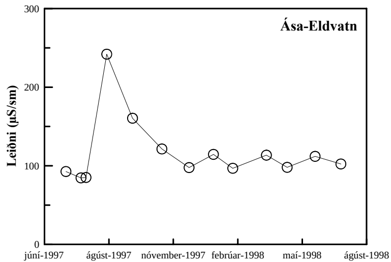
Mynd 23: Leiðni vatns í Ása-Eldvatni með tíma.
