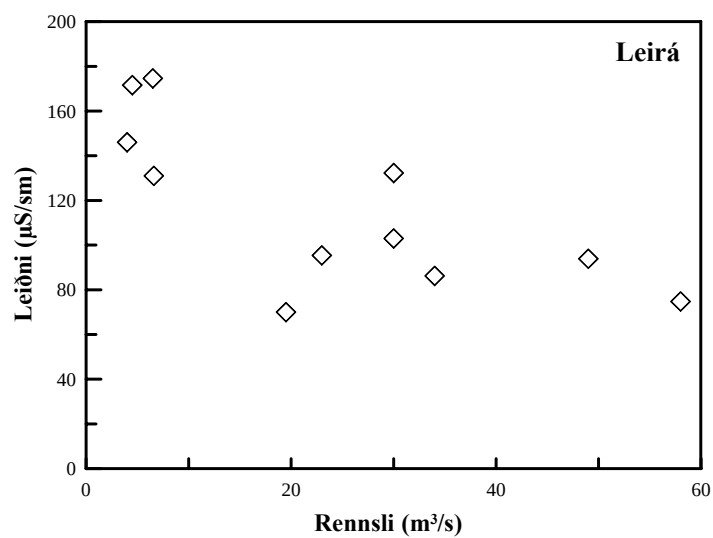
Mynd 27: Samband leiðni og rennslis í Leirá.
