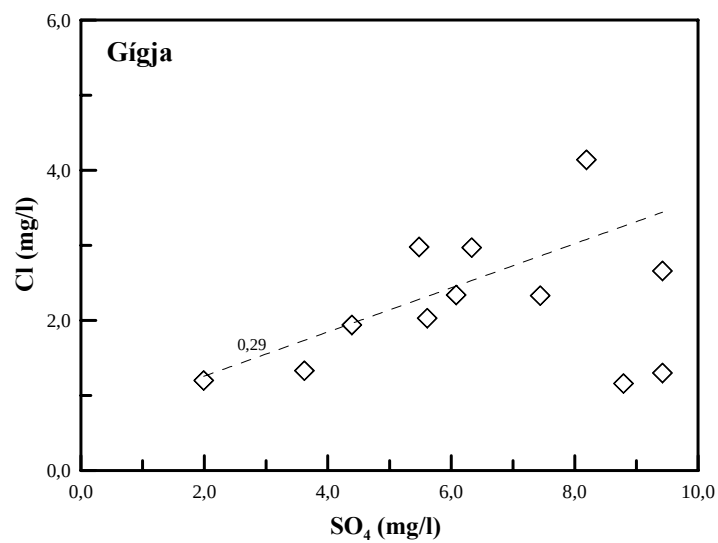
Mynd 16: Styrkur klóríðs og sulfats í Gígju.
