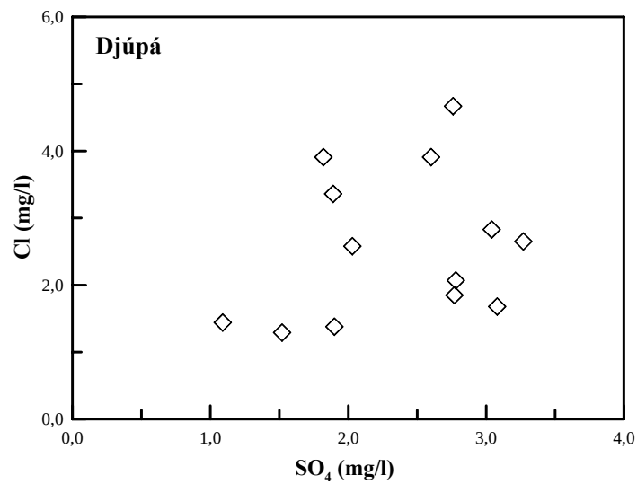
Mynd 22: Styrkur klóríðs og súlfats í Djúpá.
