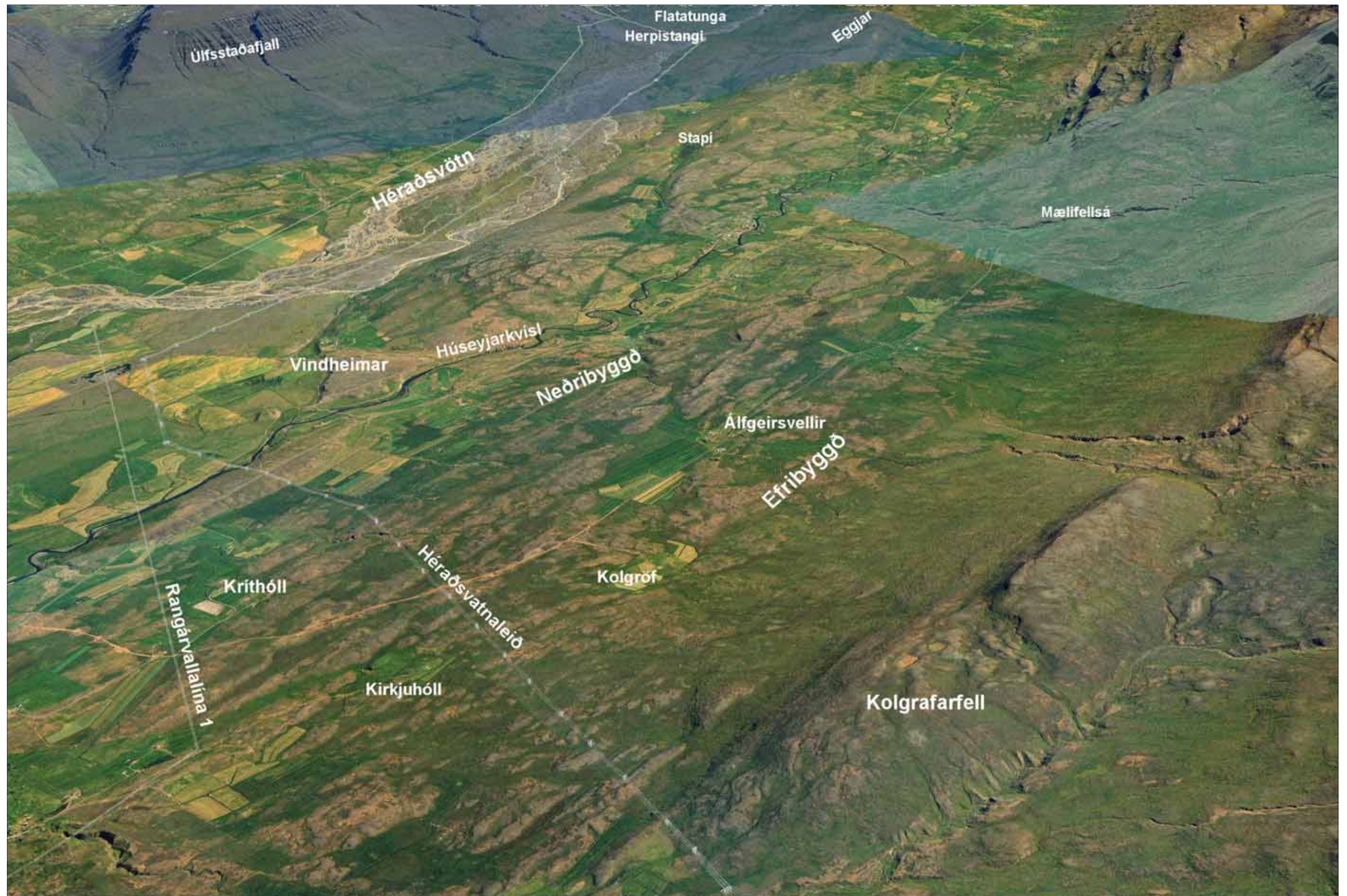
Mynd 17 Fyrirhuguð línuleið í Skagafirði, Héraðsvatnaleið.
