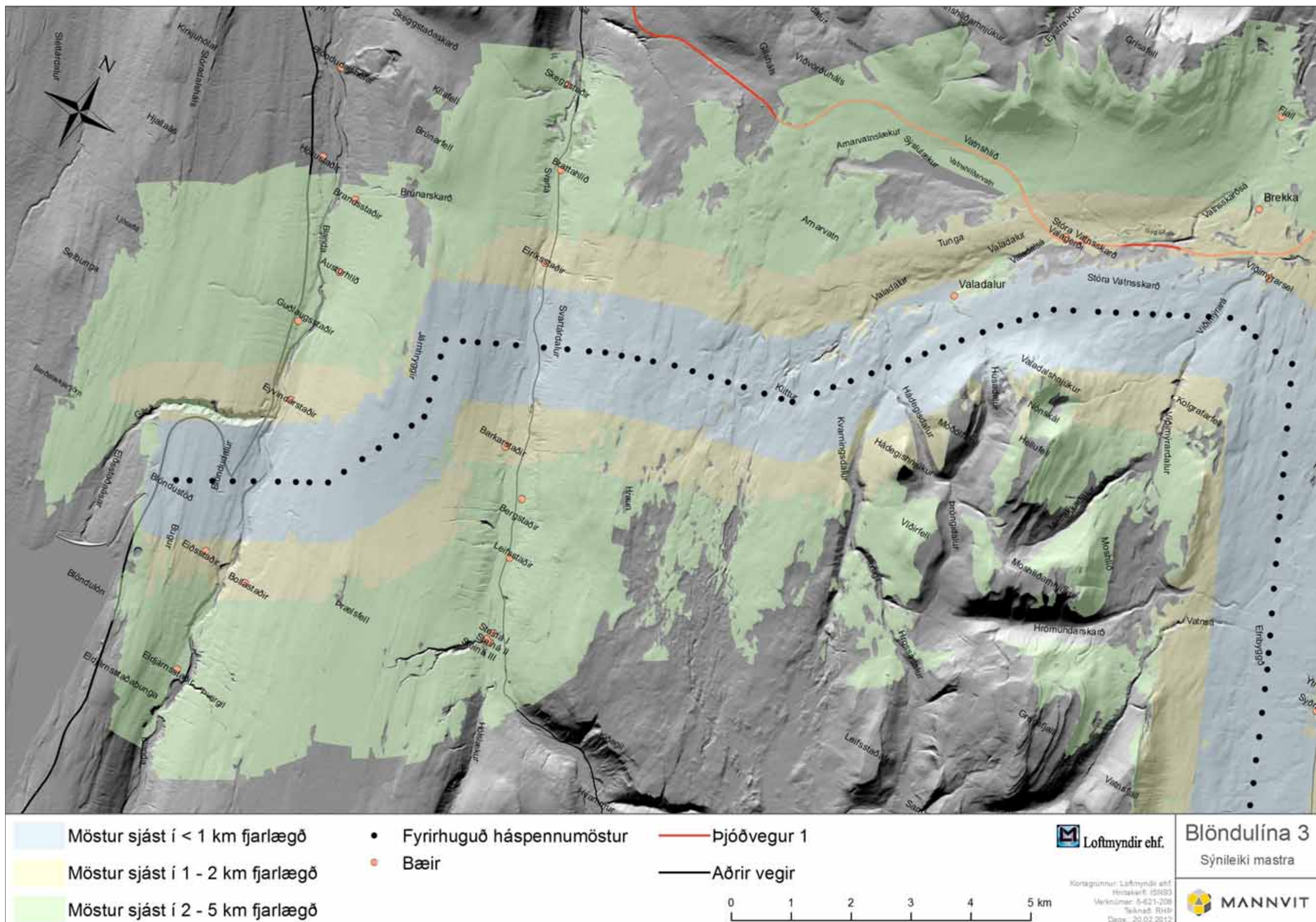
Mynd 29 Sýnileiki Blöndulínu 3 – Blönduhlíð.
