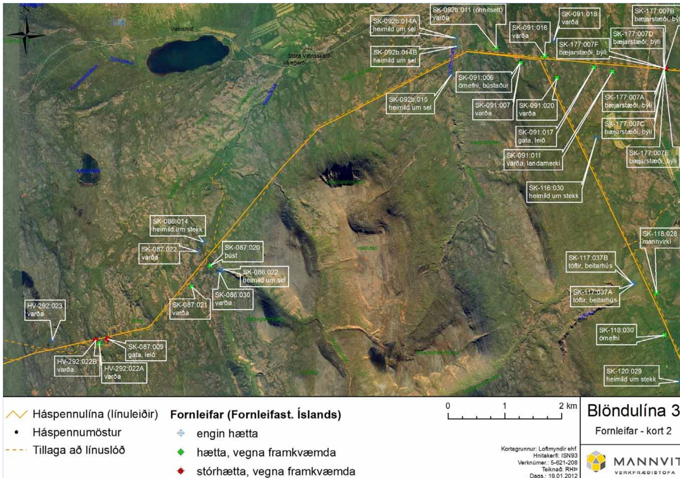
Mynd 68 Fornleifar á leið Blöndulínu 3 í hluta Húnavatnshrepps og Skagafjarðar.
