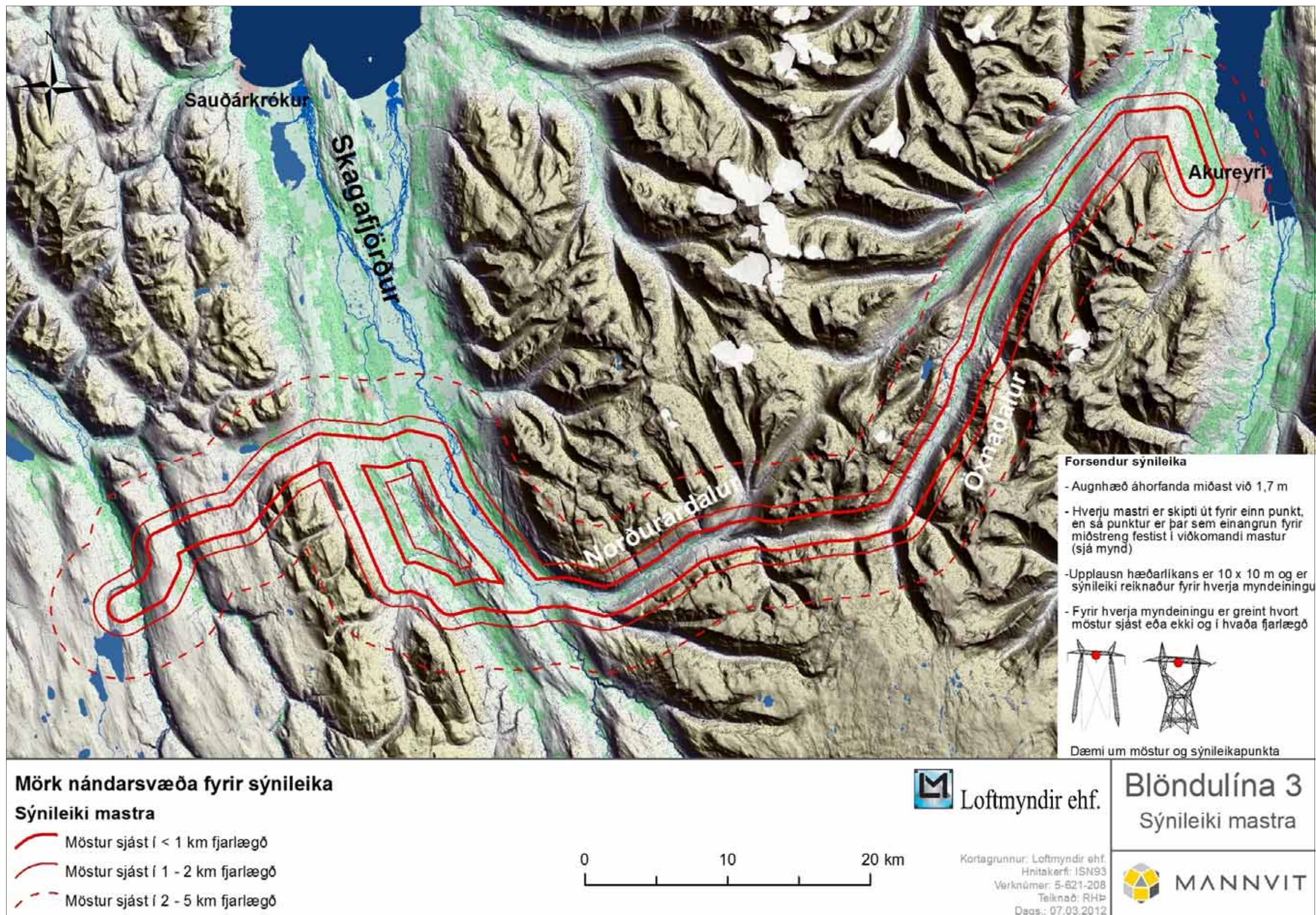
Mynd 28 Sýnileikakort fyrir Blöndulínu 3 frá Blöndustöð að Kífsá við Akureyri.
