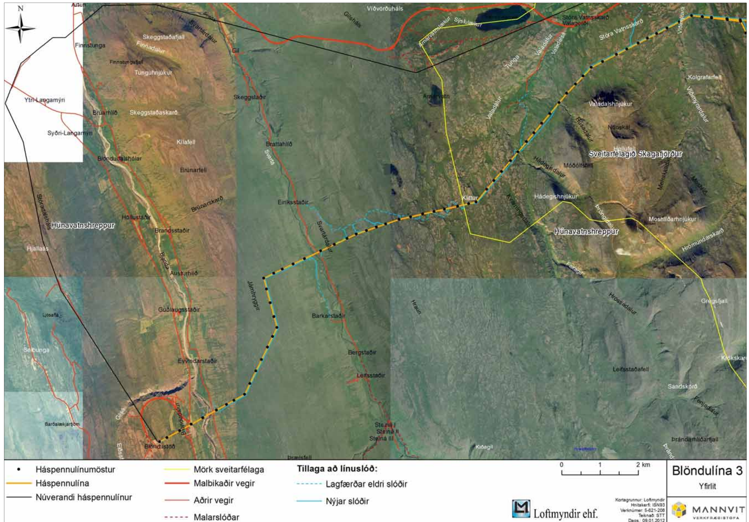
Mynd 2 Fyrirhuguð línuleið frá Blöndustöð að Kirkjuhóli í Skagafirði. Tillaga að legu slóða meðfram línunni er sýnd á myndinni.
