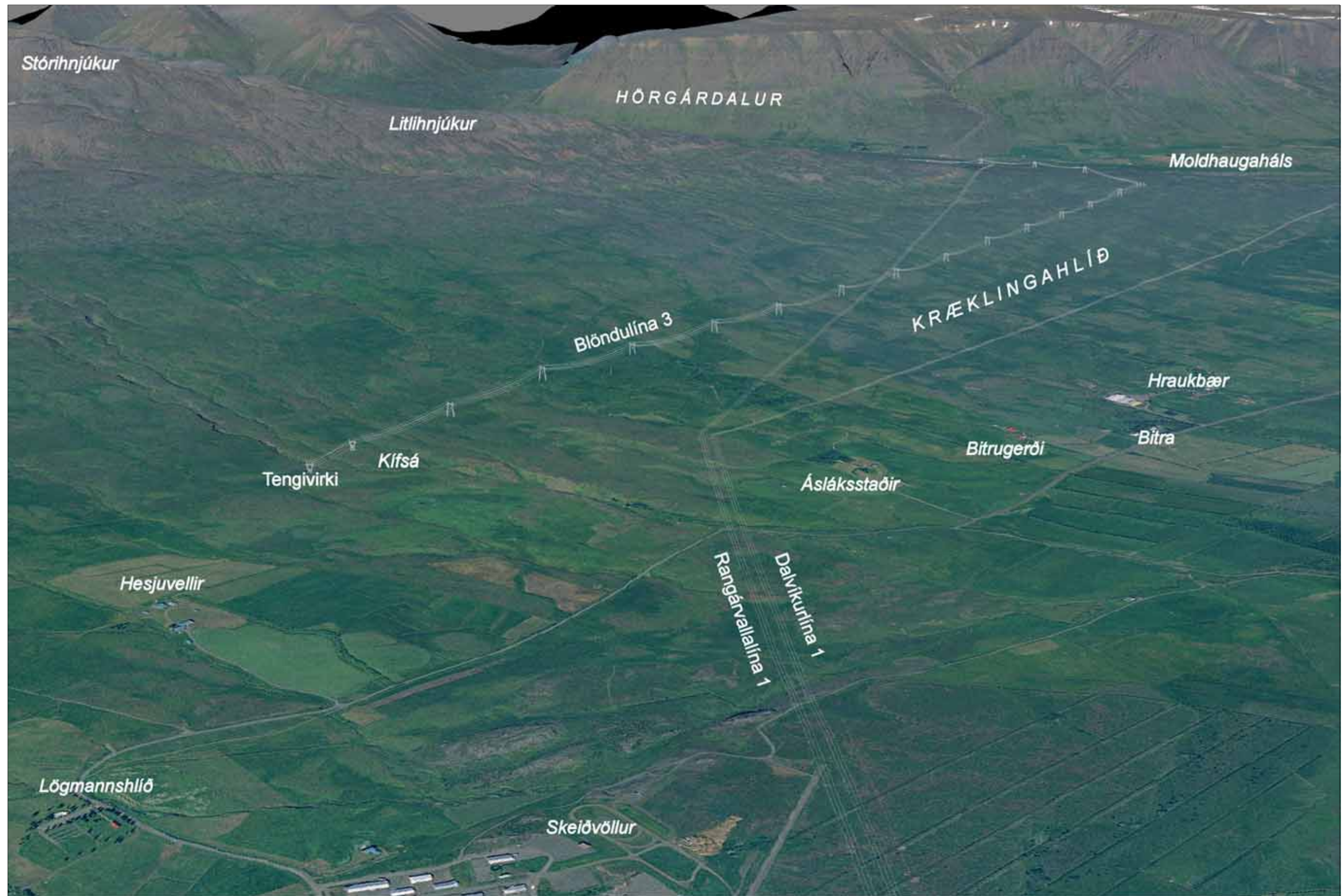
Mynd 24 Fyrirhuguð leið Blöndulínu 3 um Kræklingahlíð að tengivirki við Kífsá. Jarðstrengur mun síðan liggja frá tengivirki við Kífsá að tengivirki á Rangárvöllum (ekki sýndur á myndinni). Horft er í norðvestur.
