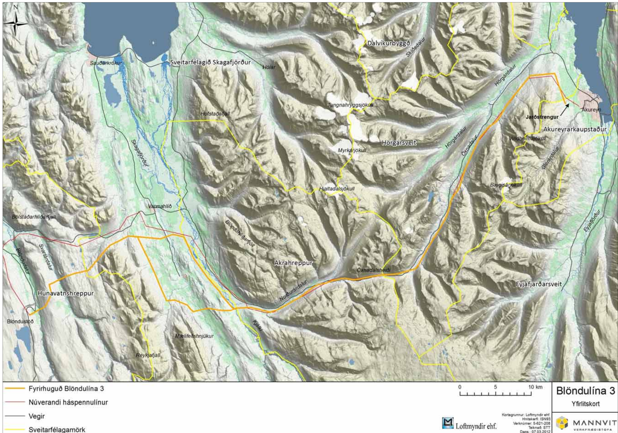
Mynd 1 Fyrirhuguð línuleið frá Blöndustöð til Akureyrar.
