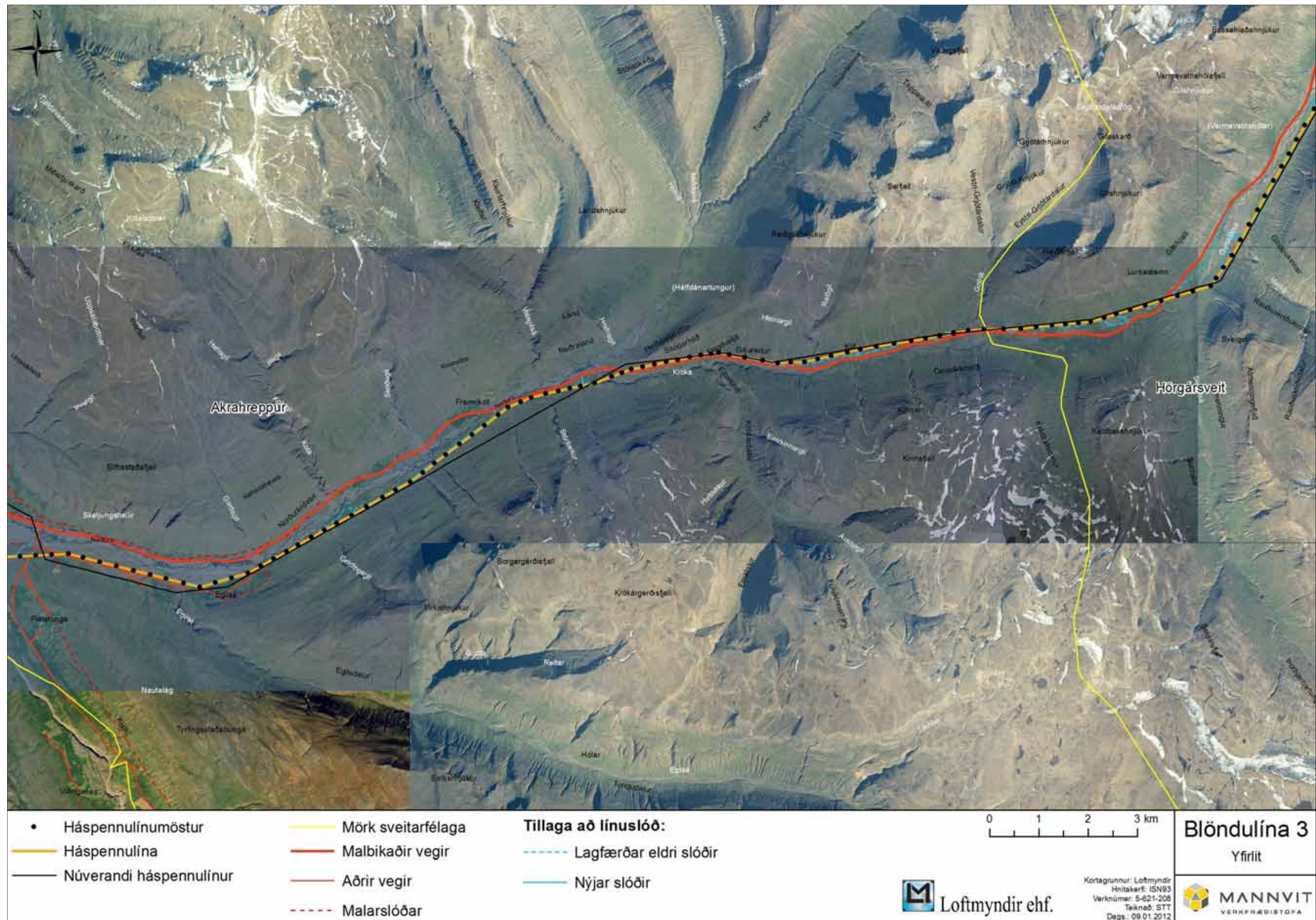
Mynd 4 Fyrirhuguð línuleið frá Herpistanga í Norðurárdal og um Öxnadalsheiði. Tillaga að legu slóða meðfram línunni er sýnd á myndinni.
