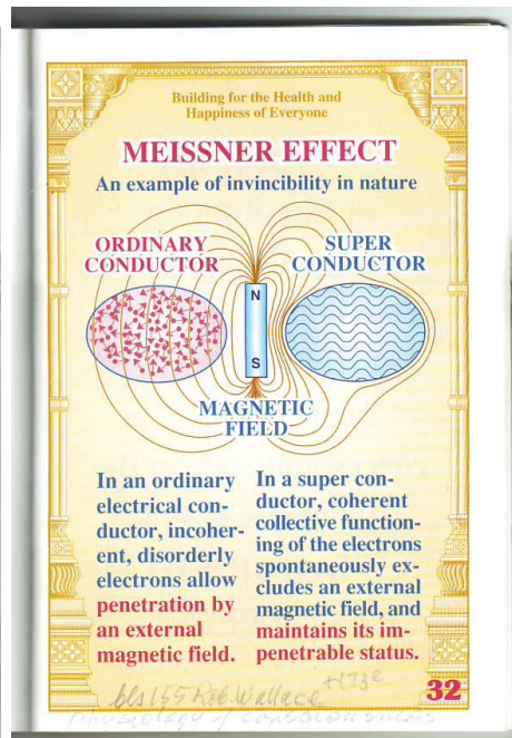
Meissner-áhrifin.
