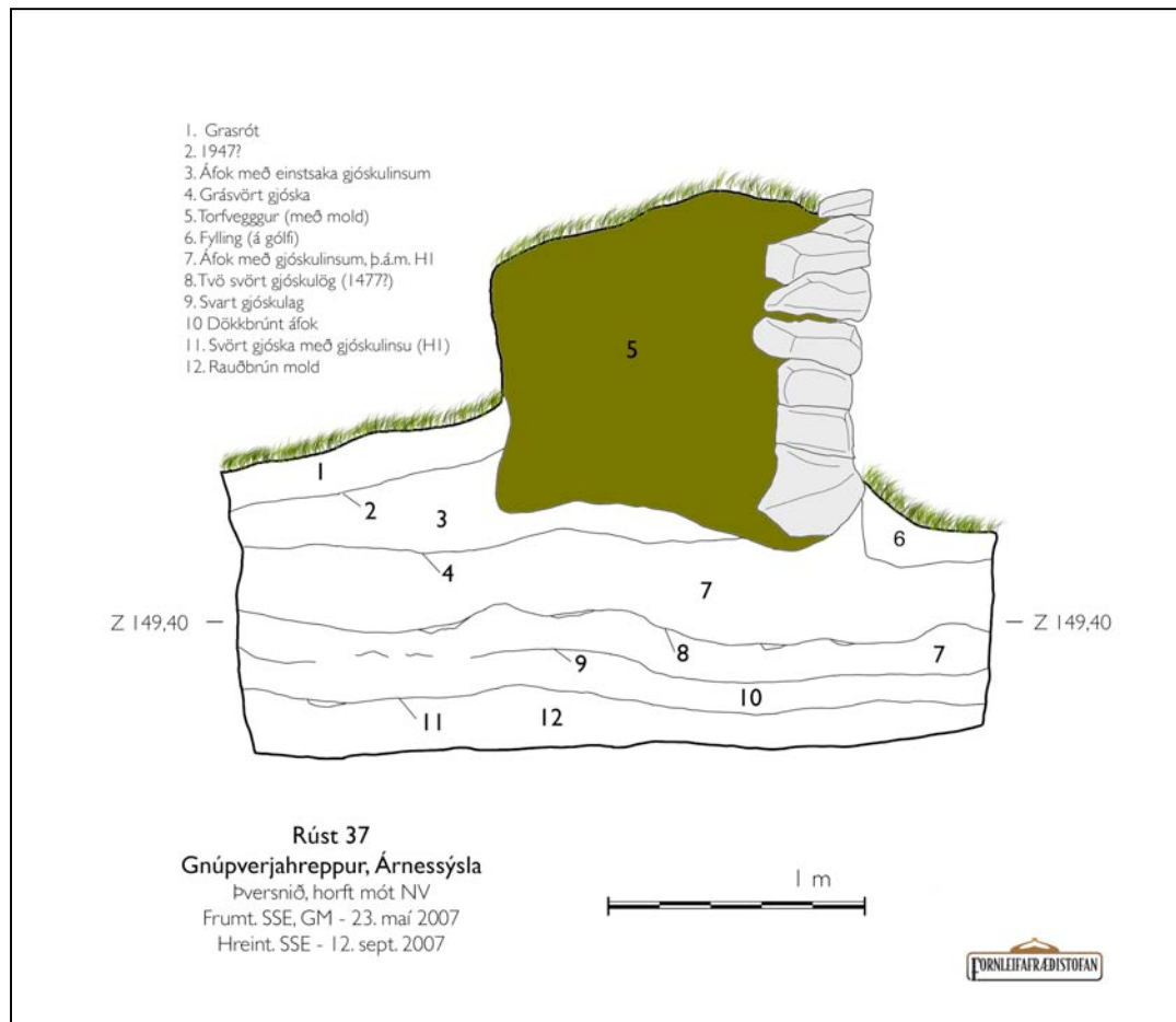
Mynd 3. Snið í vestur-langvegg rústar nr. 37. Sjá má hvernig gólf fjárhússins hefur verið grafið dálítið niður í brekkuna (sbr. lag nr. 6 á myndinni). Einnig hefur veggundirstaðan verið sléttuð áður en veggurinn var byggður.
