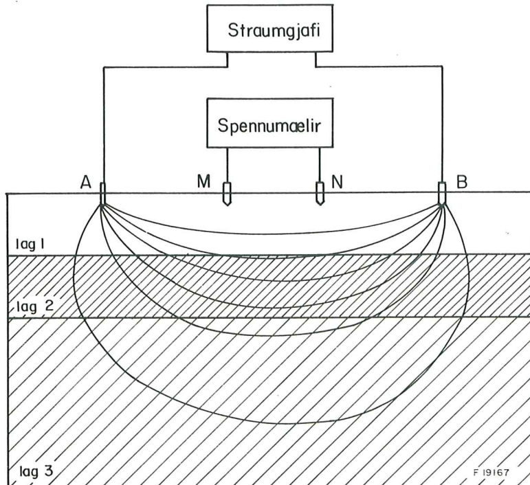
12. mynd: Fyrirkomulag straum- og spennuskauta í viðnámsmælingu, straumskautamælingu. A og B eru straumskautin. Eftir því sem lengra er á milli þeirra ná straumlínurnar til dýpri jarðлага. M og N eru spennuskaut. Unnt er að reikna eðlisviðnám jarðлага út frá mældum straum og spennu. Myndin er úr grein eftir Axel Björnsson í Náttúrufræðingnum 1980.
