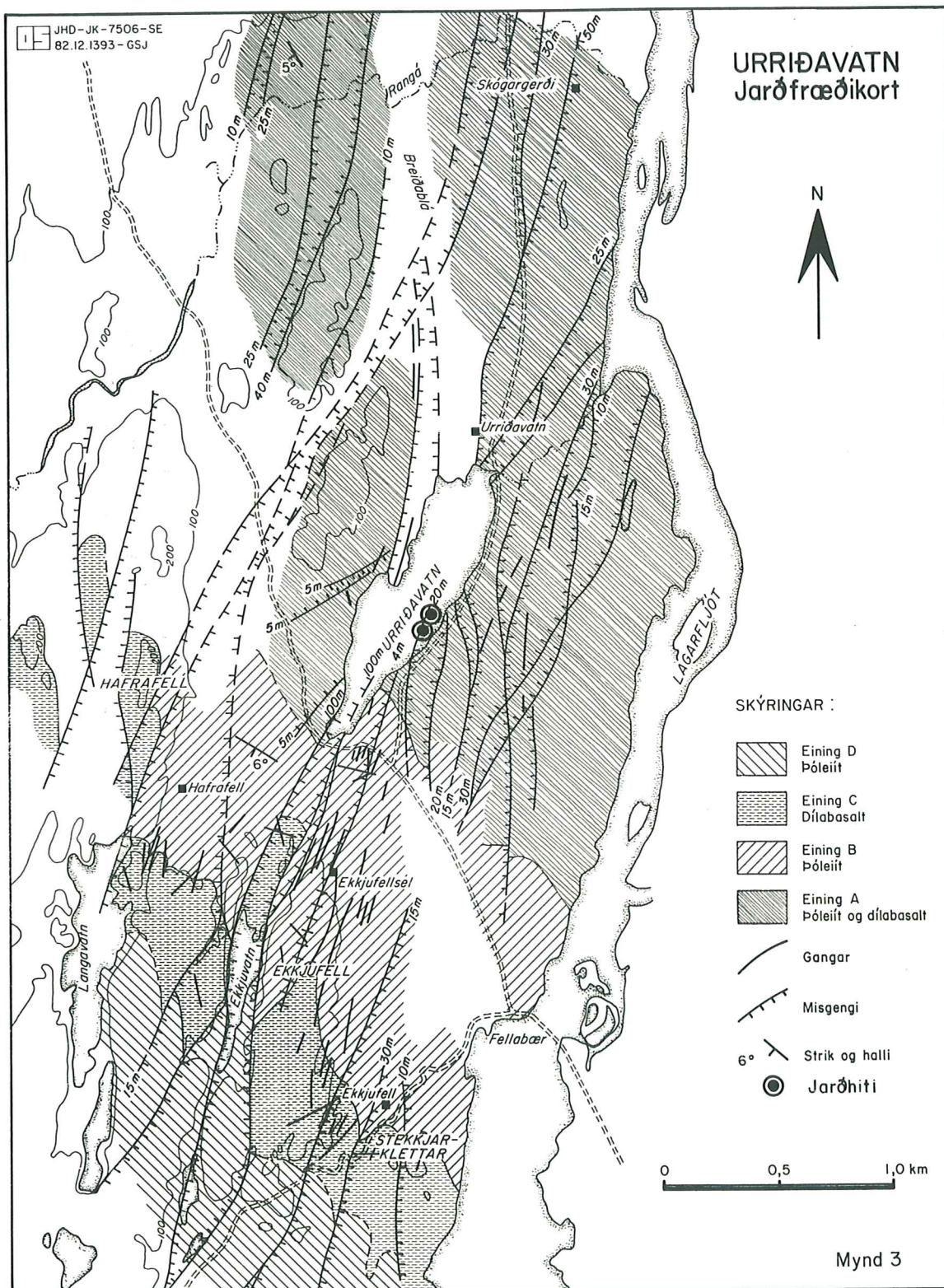
8. mynd: Jarðfræðikort af næsta nágrenni jarðhitasvæðisins í Urríðavatni. Kortið sýnir helstu jarðmyndanir á svæðinu og öll misgengi, sprungur og ganga á 10 ferkílómetra svæði. Jarðhitinn kemur upp úr vatnsbotninum og virðist vera tengdur sprungu, sem ekki sást við jarðfræðikortlagningu, en fannst í viðnámsniðmælingum. Kortið er úr skýrslu Orkustofnunar eftir Sigmundur Einarsson o.fl. frá 1983 (OS-83005/JHD-03).
