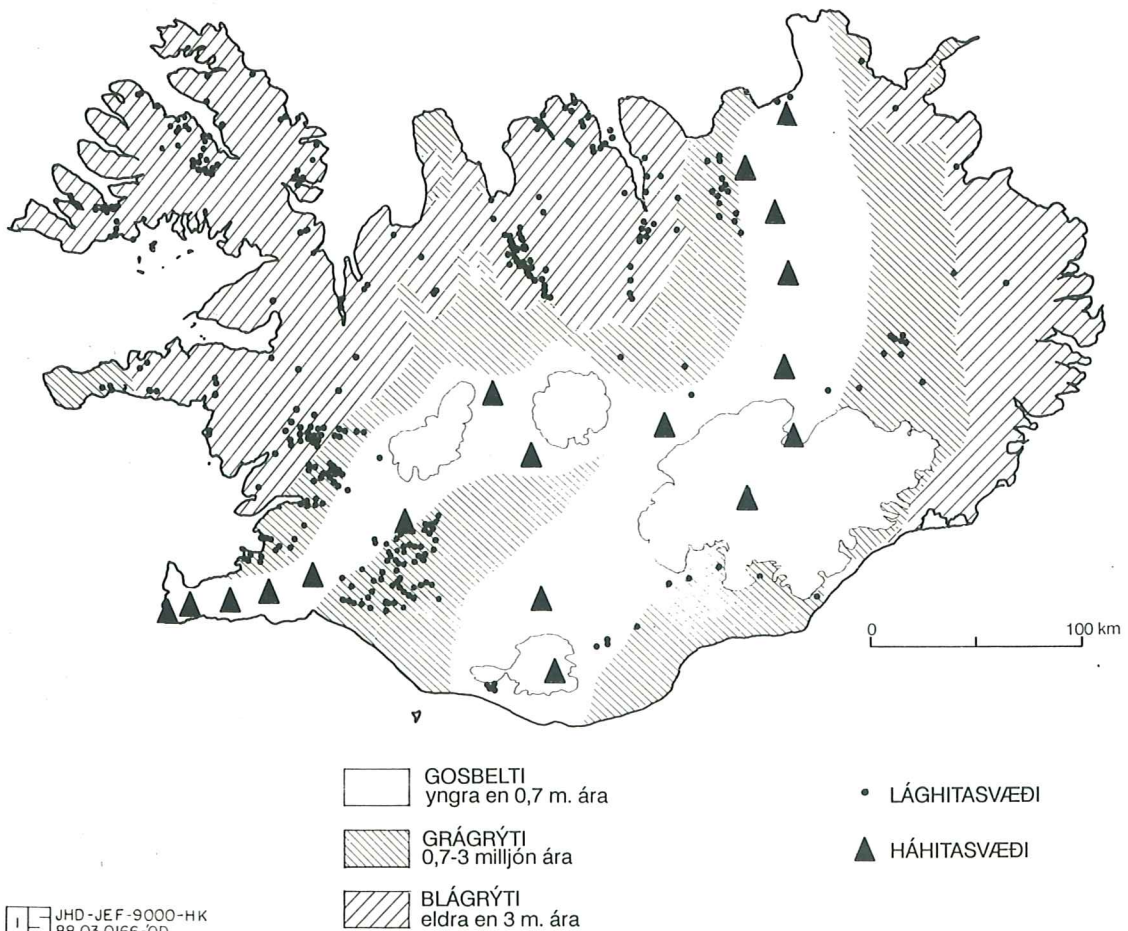
4. mynd: Jarðfræðikort af Íslandi. Óskyggða svæðið um miðbik landsins sýnir gosbeltin. Sitt hvoru megin er eldra berg, fyrst grágrýtismyndunin og austast og vestast á landinu blágrýtismyndunin. Háhitasvæðin eru einkennd með þríhyrningum, þau eru öll innan gosbeltanna. Lághitasvæðin eru sýnd með punktum. Þau öflugustu eru nálægt jöðrum gosbeltanna á Suðvesturlandi og í Þingeyjarsýslum. Mun minna er um jarðhita austan gosbeltanna heldur en vestan þeirra. Þetta ræðst af mismunandi virkni jarðskorpunnar á þessum landshlutum.
