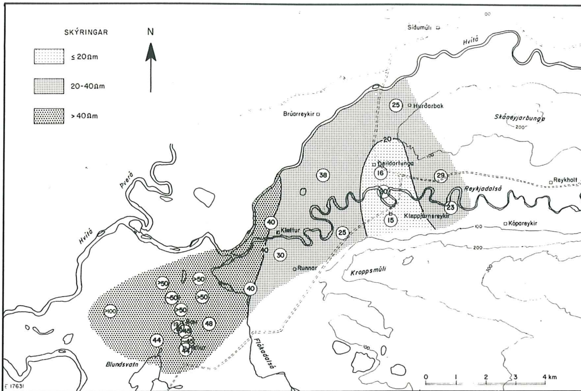
13. mynd: Eðlisviðnám jarðlaga á 800 m dýpi í vestanverðum Reykholtstalur í Borgarfirði. Hringirnir sýna staðsetningu viðnámsmælinga og tölurnar eðlisviðnám á 800 m dýpi. Áberandi lágvíðnámssvæði er umhverfis jarðhitastaðina við Deildartunga og Kleppjárnreyki. Orsök þess er vatnsgengt berg og hár hiti. Myndin er úr skýrslu Orkustofnunar eftir Lúðvík Georgsson o.fl. frá 1978 (OS-JHD-7856).
