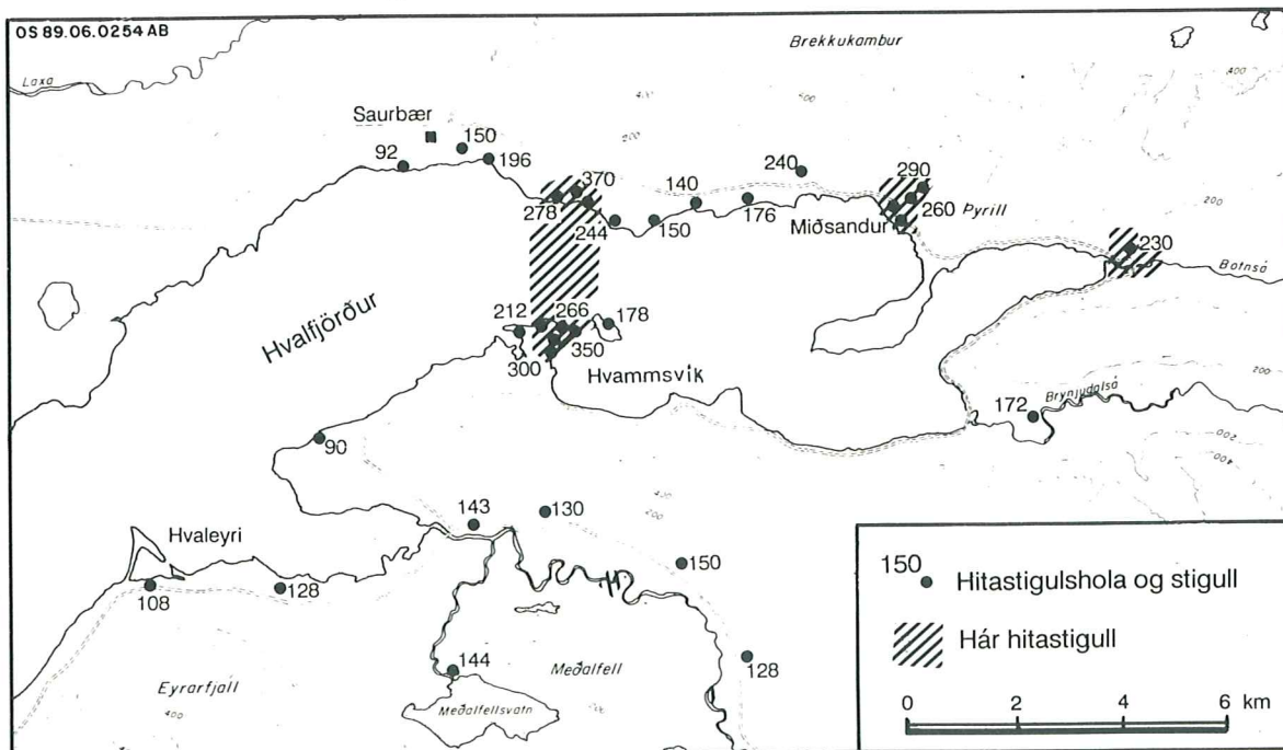
17. mynd: Hitastigull í grunnnum borholum á Hvalfjarðarströnd og við sunnanverðan Hvalfjörð. Svæðisbundinn hitastigull er um eða yfir 100 °C á kílómetra. Övenju hár hitastigull mældist á nokkrum stöðum. Athyglisverðast er frávik, sem virðist teygja sig undir fjörðinn á mótis við Hvammsvík. Niðurstöðurnar voru notaðar til þess að staðsetja djúpa borholu austan Saurbæjar og gaf hún góðan árangur eða yfir 20 l/sek af 80 °C heitu vatni. Þetta er á svæði, þar sem enginn jarðhiti er á yfirborði. Myndin er úr erindi Kristjáns Sæmundssonar á ársfundri Orkustofnunar 1989.
