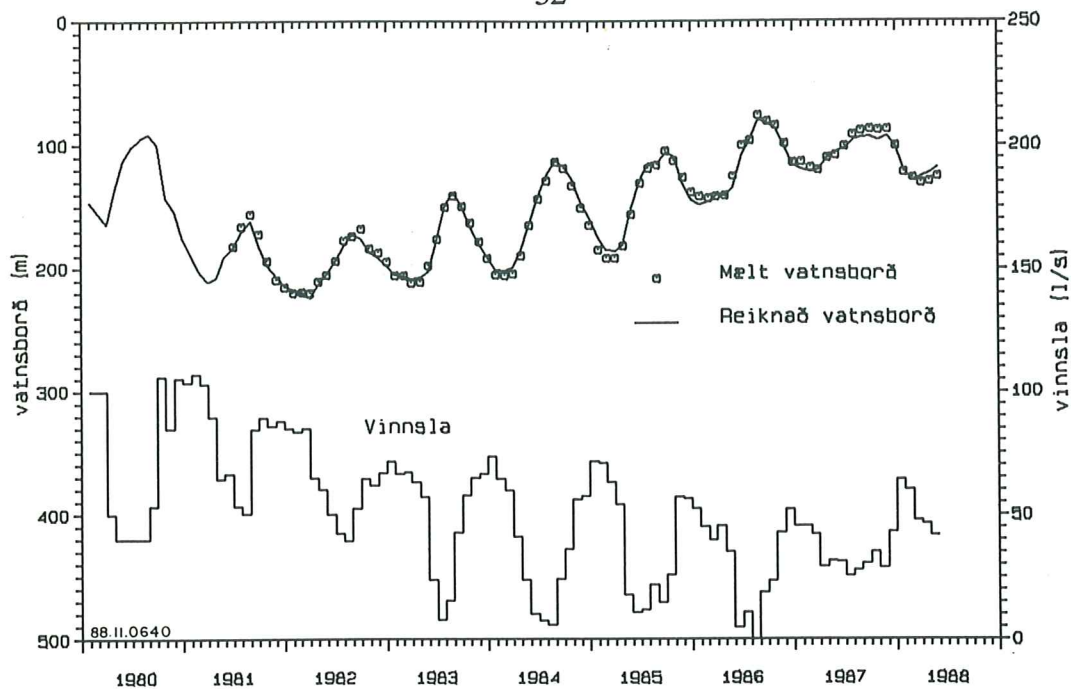
28. mynd: Vinnslusaga jarðhitasvæðisins að Laugalandi í Eyjafirði. Neðri hluti myndarinnar sýnir vatnsvinnslu úr jarðhitakerfinu á árunum 1980 til 1988, mælt í lítrum á sekúndu. Punktarnir á efri hlutanum sýna mælt vatnsborð, sem sveiflast í takt við vinnsluna. Heildregna línan í gegnum mældu punktana sýnir vatnsborð, reiknað með hermílkani, sem lagað hefur verið að mældu gögnunum. Myndin er úr skýrslu Orkustofnunar eftir Guðna Axelsson o.fl. frá 1988 (OS-88052/JHD-10).
