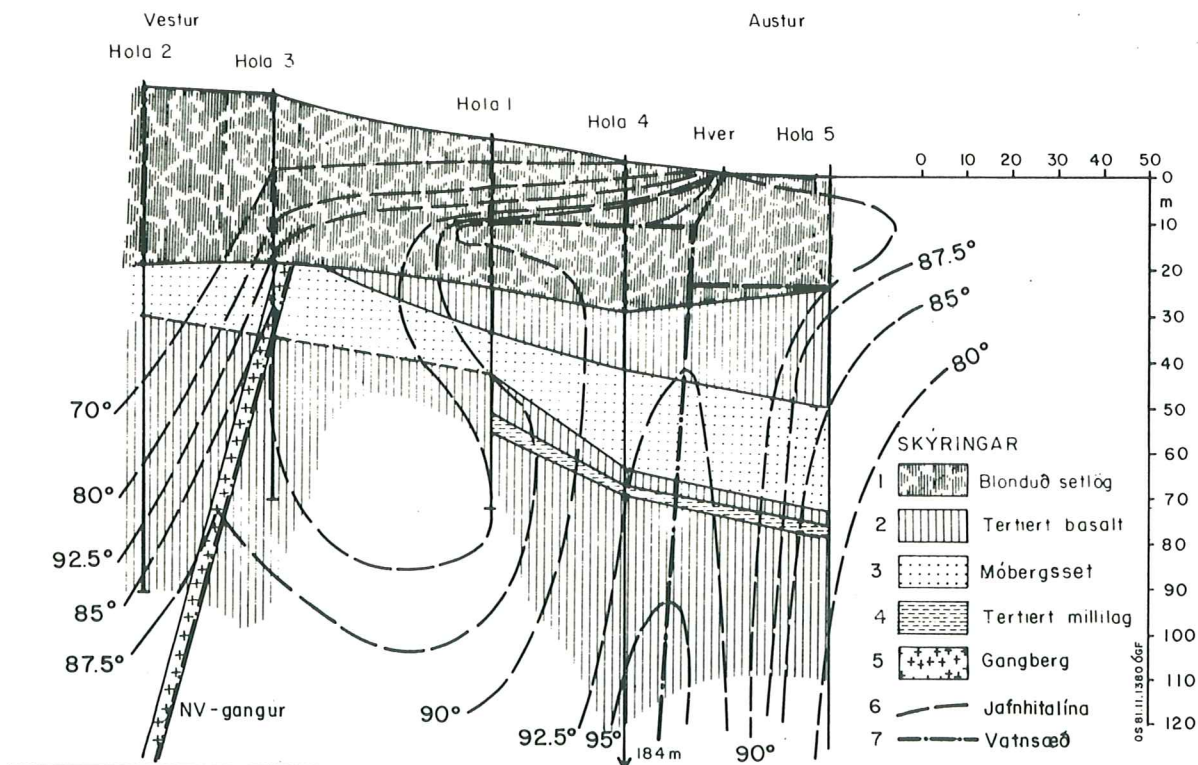
21. mynd: Jarðlagasnið af jarðhitasvæðinu að Reykjum í Fnjóskadal. Sýnd eru jarðlög samkvæmt svarfgreiningu, hitadreifing samkvæmt hitamælingum í borholum svo og berggangar og vatnsleiðandi sprungur. Myndin er úr skýrslu Orkustofnunar eftir Ólaf Flóvenz o.fl. frá 1982 (OS-82050/JHD-08).
