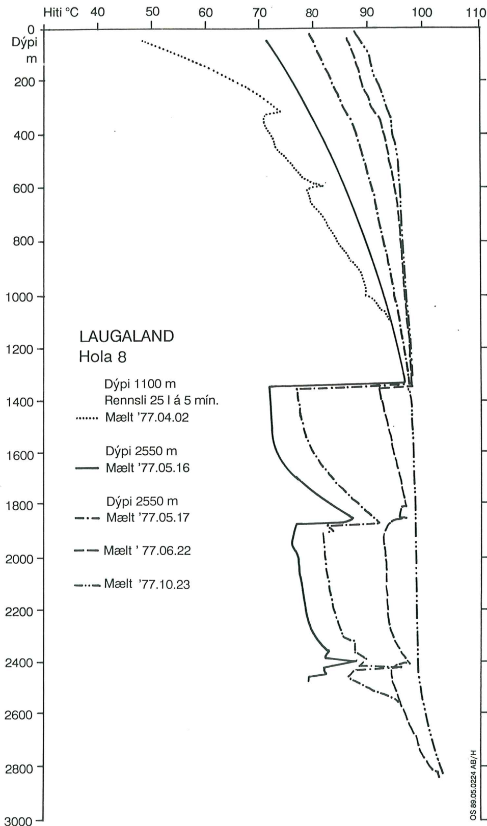
23. mynd: Hitaferlar úr borholu númer 8 að Laugalandi í Eyjafirði. Fyrsti ferillinn er mældur þegar holan var 1100 m djúp og sjást á honum vatnsæðar á 320 og 590 m dýpi. Næstu tveir ferlar eru mældir þegar holan var orðin 2550 m djúp og þar sjást æðar á 1340 m, 1860 m og 2400 m dýpi, en efti æðarnar sjást ekki vegna rennslis að neðan. Ferillinn lengst til hægri er mældur þegar holan hefur hitnað upp eftir borun. Mælingarnar sýna að hiti í vatnsæðum í holunni er á bilinu 75-100 °C. Fyrir neðan 2400 m vex hitastig ört, sem gæti bent til þess að hringrás jarðhitakerfisins nái ekki neðar. Svæðisbundinn hitastigull í Eyjafirði utan jarðhitasvæða er 60 °C/km. Þetta sýnir að hræring vatns í jarðhitakerfinu hefur hitað upp bergið ofan við 1600 m dýpi en kælt berg þar fyrir neðan. Myndin er úr skýrslu Orkustofnunar eftir Axel Björnsson o.fl. frá 1979 (OS-JHD-7827).
