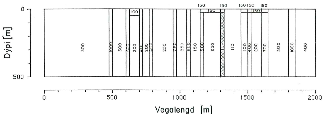
14. mynd: Líkan er sýnir eðlisviðnám í jarðlögum á sniði sem liggur austur vestur í gegn um jarðhitasvæðið í Urriðavatni. Líkanið einkennist af lóðréttum bergmyndunum (berggöngum), sem hafa hátt viðnám. Ein myndun, sem er skyggð á myndinni, hefur áberandi lágt viðnám. Það er líklegast sprunga, sem er meginleiðari heita vatnsins. Sniðið er unnið upp úr viðnámsmælingum og voru niðurstöðurnar notaðar til þess að staðsetja aðal vinnsluhölu hitaveitunnar á staðnum. Myndin er úr skýrslu Orkustofnunar eftir Sigmund Einarsson o.fl. frá 1983 (OS-83005/JHD-03).
