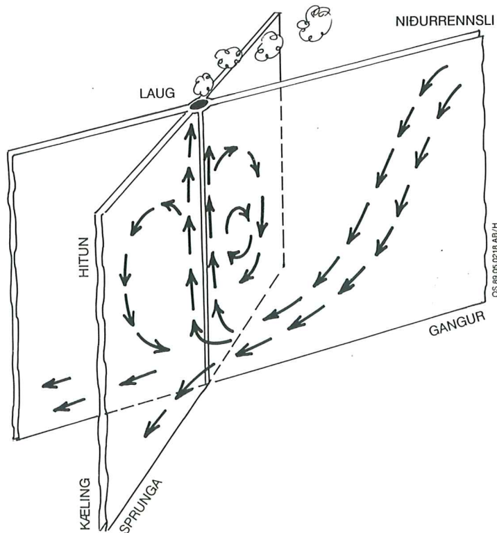
6. mynd: Lághitasvæði eru gjarnan tengd tveimur sprungukerfum með mismunandi stefnu. Þar sem sprungurnar skerast er lektin best og heita vatnið leitar þar upp til yfirborðs.
