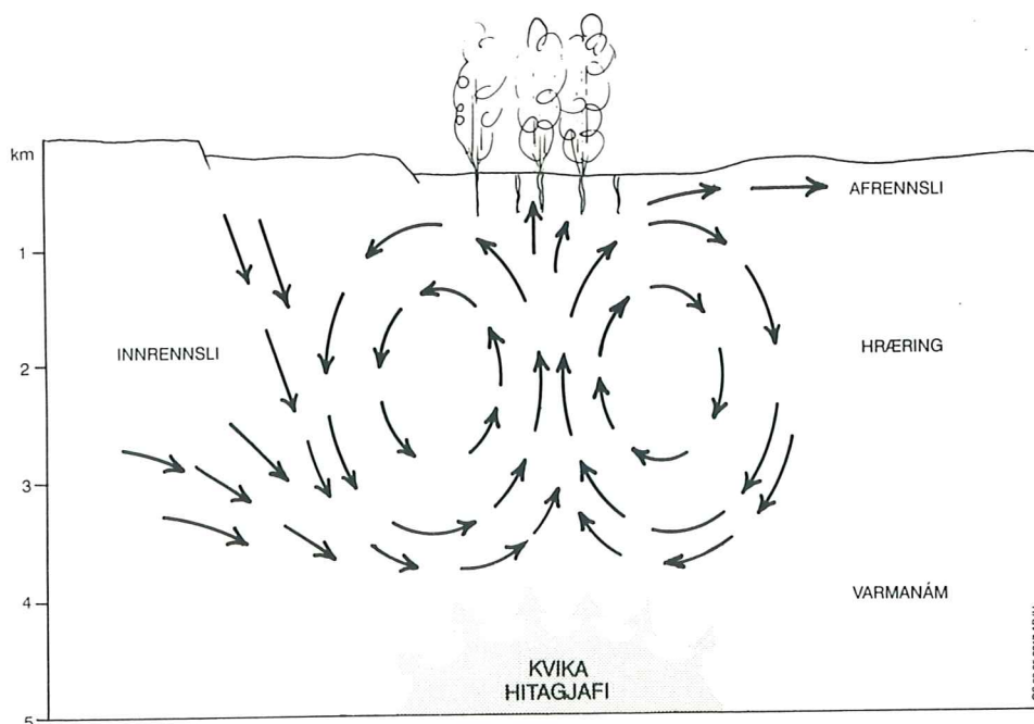
7. mynd: Einfölduð mynd af háhitasvæði. Háhitasvæði myndast við staðbundna hringrás vatns í sprungnu bergi yfir kvikuhólfi eða kólnandi innskoti sem er á fárra kílómetra dýpi í jarðskorpunni.
