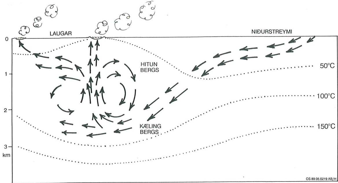
5. mynd: Líkan af lághitasvæði. Lághitasvæðin myndast við hringrás vatns í sprungum og brotnu bergi. Kalt regn og grunnvatn seitlar djúpt niður í jarðskorpuna. Þar hitnar það í heitu bergi, og stígur síðan upp til yfirborðs eftir sprungum og myndar hverir og laugar. Hringrás vatnsins nemur varma úr neðri hluta skorpunnar, sem kólnar við það og flytur varmann upp í efri jarðlög. Afl lághitasvæða er einkum háð lekt jarðlaga og hitastigli.
