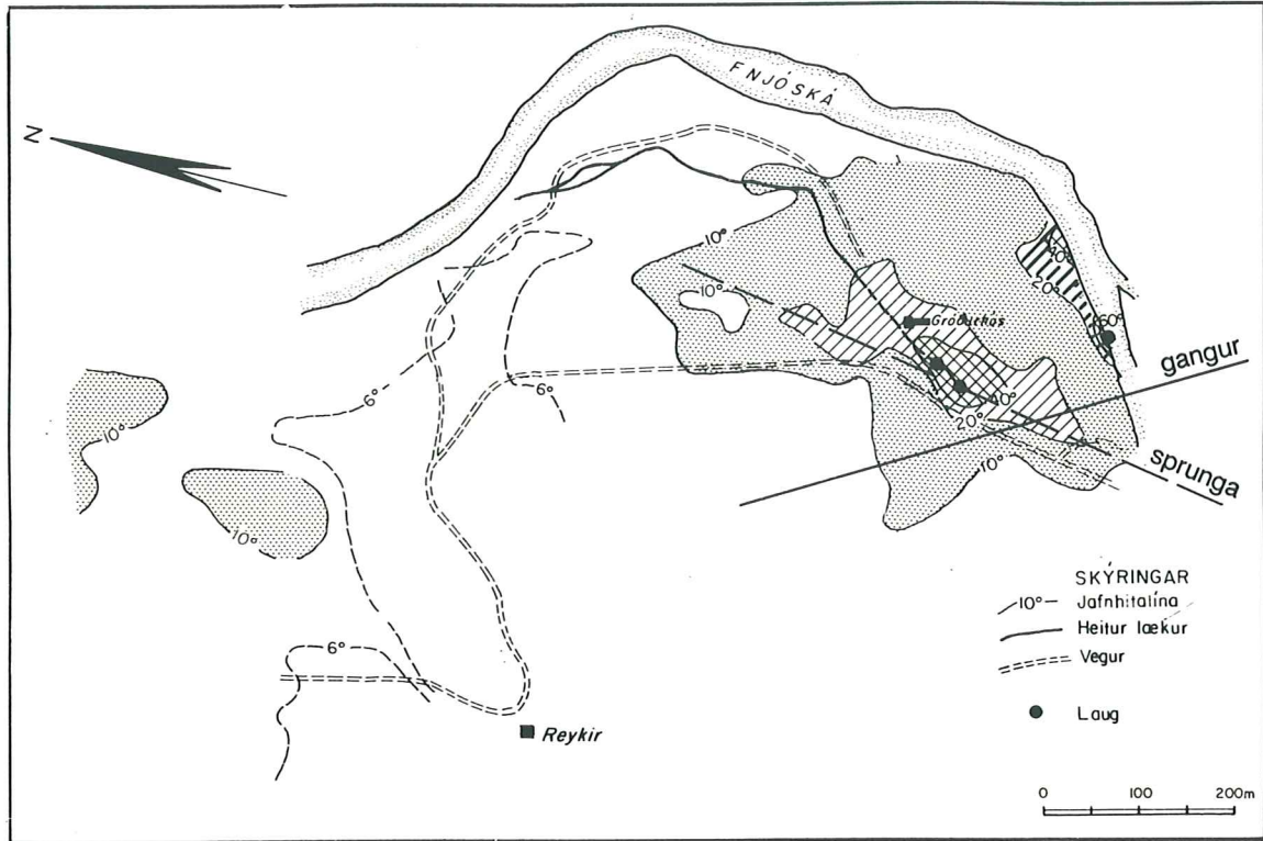
11. mynd: Hitastig í jarðvegi á 50 sm dýpi við Reyki í Fnjóskadal. Hiti er hæstur eða 40 °C næst laugunum og á bökkum Fnjóskár austan laugasvæðisins. Hitafrávikidið við laugarnar er aflangt í norður suður stefnu, og bendir það til þess að uppstreymi heita vatnsins sé tengt sprungu með þeirri stefnu. Inn á myndina er einnig teiknaður gangur sem kom fram í mælingum. Myndin er úr skýrslu Orkustofnunar eftir Ólaf Flóvenz frá 1980 (OS-80009/JHD-05).
