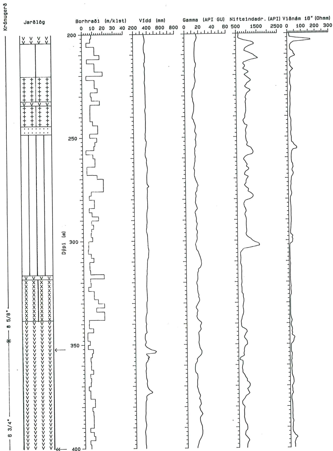
20. mynd: Jarðlög og borholumælingar á 200 - 400 m dýpi úr holu númer 1 á Bakka í Ölfusi. Lengst til vinstri á myndinni er sýnd krónustærð og jarðlög samkvæmt svarfgræiningu. Mismunandi jarðlög eru einkennd hvert með sínu tákni. Þá kemur dýptarskali og borhraði, mældur í metrum á klukkustund. Borhraðinn ræðst einkum af hörku bergsins. Næst er sýnd vidd holunnar, þá gammageislun úr berginu, en með henni má greina súr berglög (líparít). Lengst til hægri er nifteindamæling og viðnám í holunni, en hvort tveggja er mælikvarði á vatnsinnihald bergsins.
