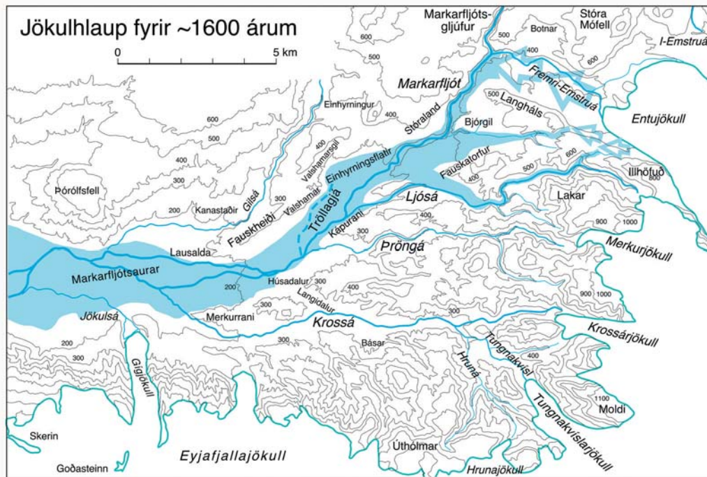
Mynd 8d. Líklegustu leiðir blaups fyrir um 1600 árum. Það var stórblaup (stærðarflokkur 4) en náði ekki upp á hjallana meðfram Fauskheiði. Lega jökuljaðra var önnur þá en nú. Örvar (ófylltar) tákna líklegar rennislíleiðir undir, meðfram eða á jökli.
