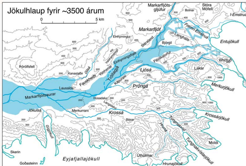
Mynd 8b. Líklegustu leiðir hlaups fyrir um 3500 árum. Það var hamfarablaup (stærðarflokkur 5). Lega jökuljaðra var önnur þá en nú. Örvar (óþylltar) tákna líklegar rennislíðir undir, meðfram eða á jökli.
