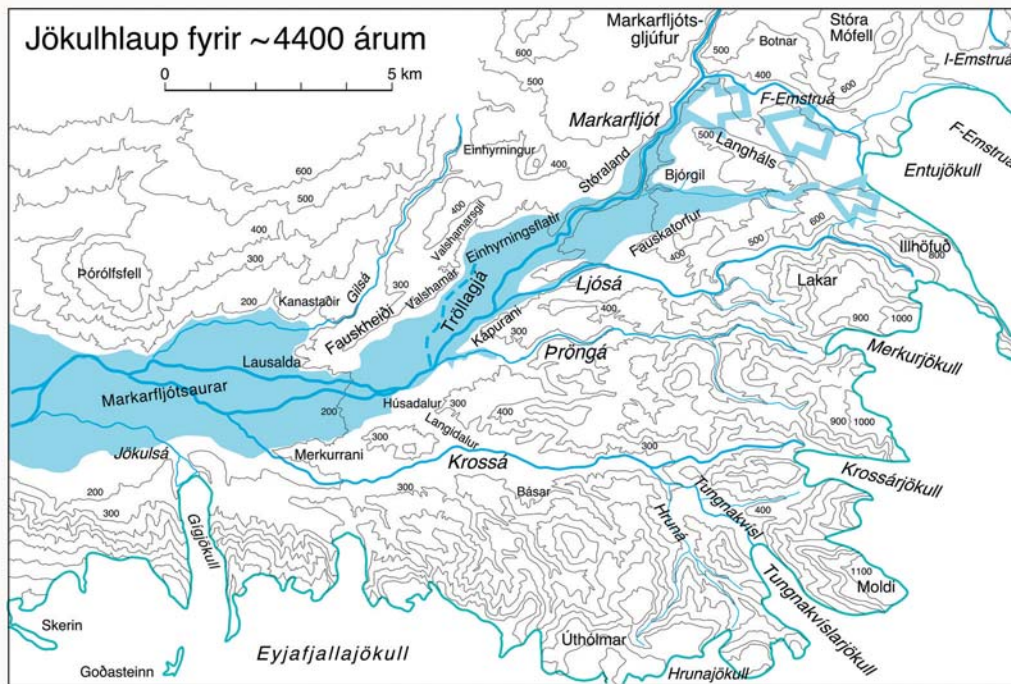
Mynd 8a. Líklegustu leiðir blaups fyrir um 4400 árum. Það var hamfarablaup (stærðarflokkur 5) og fór hærra upp í blíðar í Fauskheiði og Kápurana en önnur foröguleg blaup. Lega jökuljæðra var önnur þá en nú. Örvar (ófylltar) tákna líklegar rennslisleiðir undir, meðfram eða á jökli.
