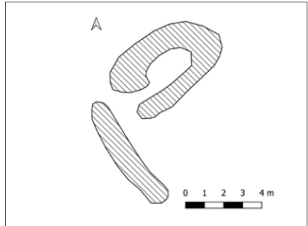
Uppmæling af stekk ÁR-247:008.
