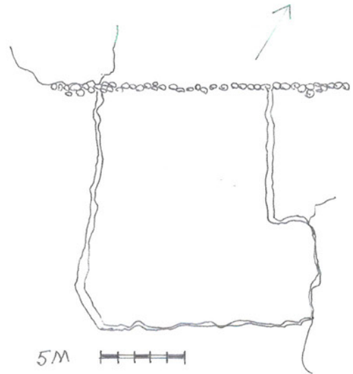
Teikning matjurtagarðurinn
