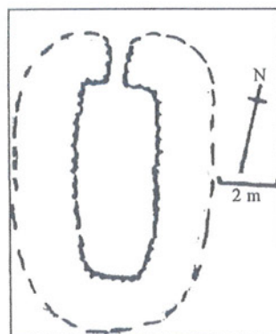
Teikning: Fornleifakönnun 2001.
