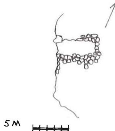
Teikning, tóftin.
