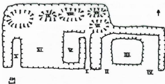
Mynd 2. Uppdráttur af bæjarhúsum, 305-01. I: bæjargöng, II: skemma, III: hlaða, IV: fjós, V: baðstofa, VI: búr, VII: hlóðaelldhús, VIII, IX: heygarður, X: hesthús/fjós, XI: garður og hlandfor þegar X var fjós.
