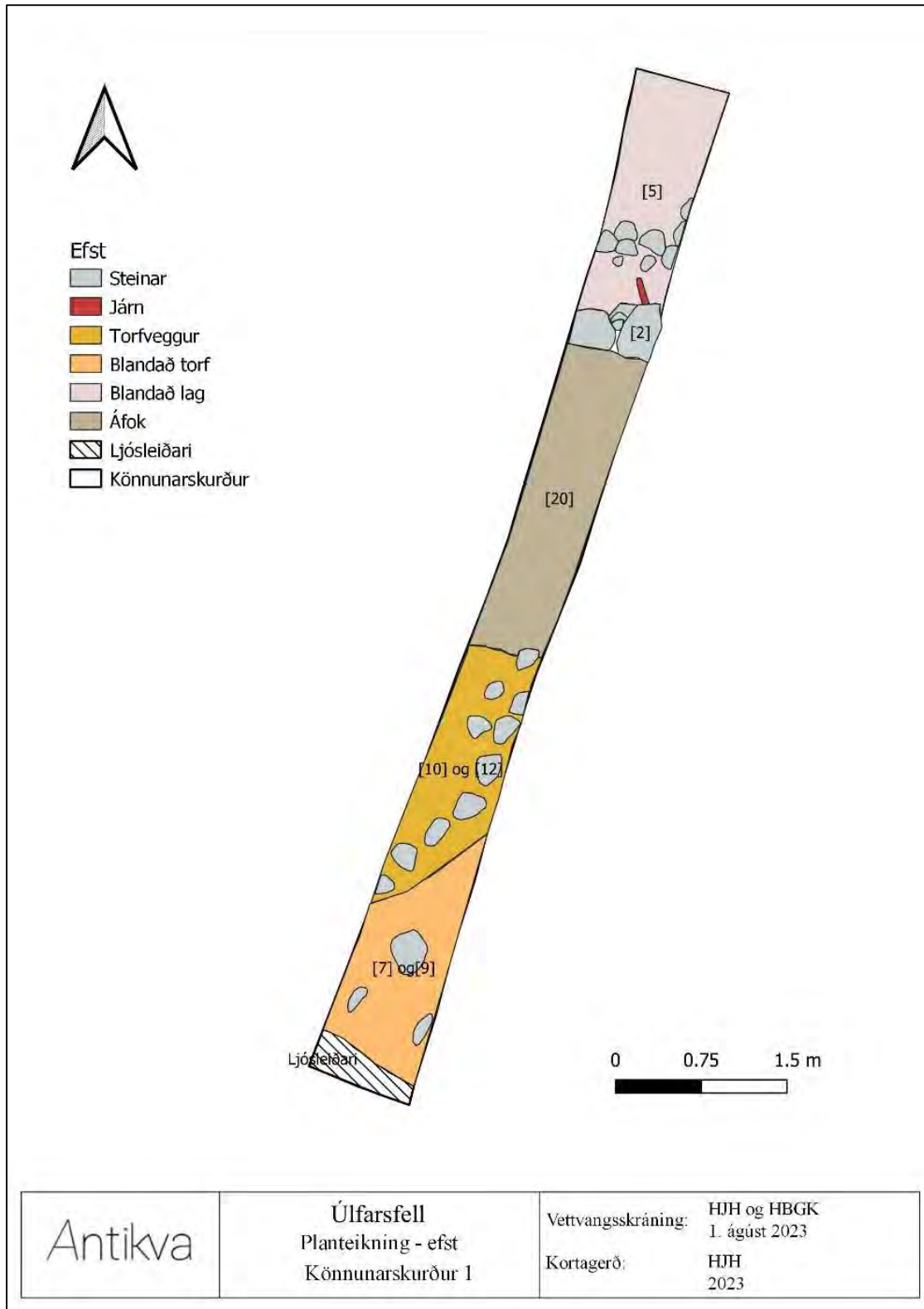
Teikning 1. Efstu mannvistarlögin sem komu í ljós.
