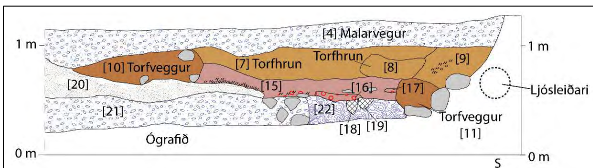
Teikning 4. Austursnið, suðurendi.
