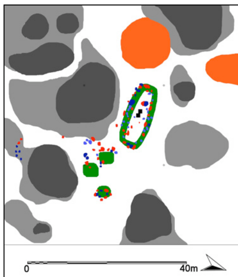
Mynd 9 og 10. Myndin til vinstri sýnir segulmæling af Vogu og nánasta umhverfi. Til hægri má sjá túlkun niðurstaðna jarðsjármælinganna. Grænt sýnir rústir, appelsínurautt sýnir hugsanlegar rústir, rautt og blátt sýnir sennilega grjótt eða grjóthleðslur. Mælingar: Tim Horsley, Bradford University..
