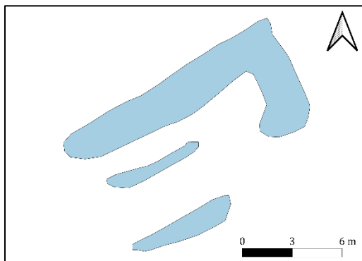
Mynd 79. Uppmæling af fjárhúsi 3121-051.
