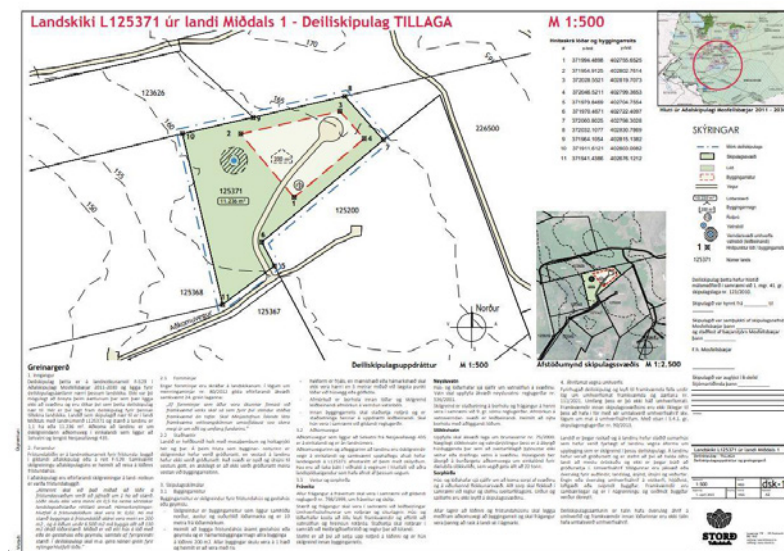
Mynd 1 – Skipulagsuppráttur unninn af Storð teiknistofu dagsettur 01.04.2023.
