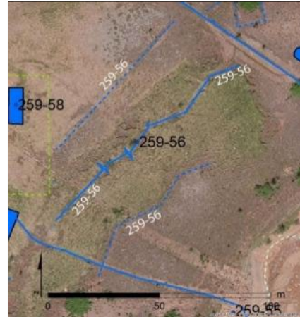
Mynd 33. Niðurgröftur (259-56), teiknað eftir uppmælingu (heil lína) og loftmynd (brotalína). 41
