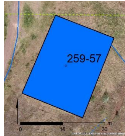
Mynd 36. Ummál steypuleifa (259-57).
