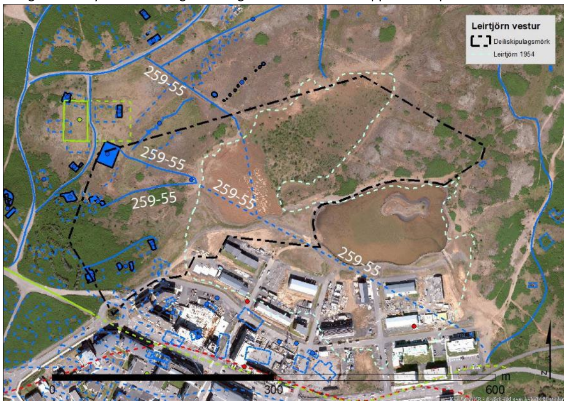
Mynd 24. Þrjár lagnaleiðir (259-55) sem lágu frá kampinum að bakka Leirtjarnarinnar tvær sameinuðust í eina sem lá áfram til suðausturs að affalli en sú nyrsta sameinaðist henni um 90 m frá bakkanum.
