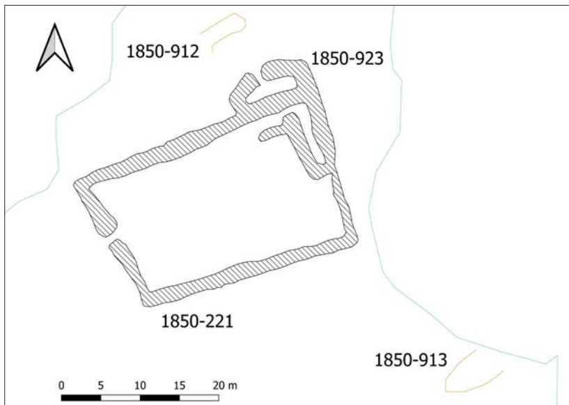
Uppmælingar af minjum við Torfdal 1850-923.
