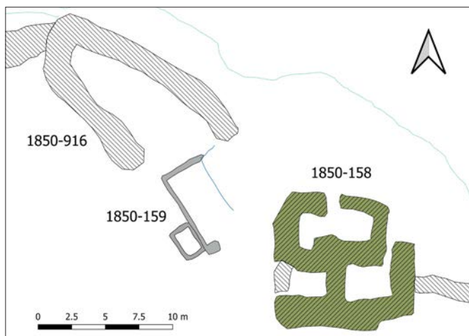
1850-158: Uppmæling af verbúðinni og nálægum minjum.
