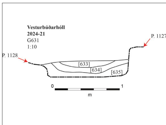
Mynd 32. Sníðteikning [631].
