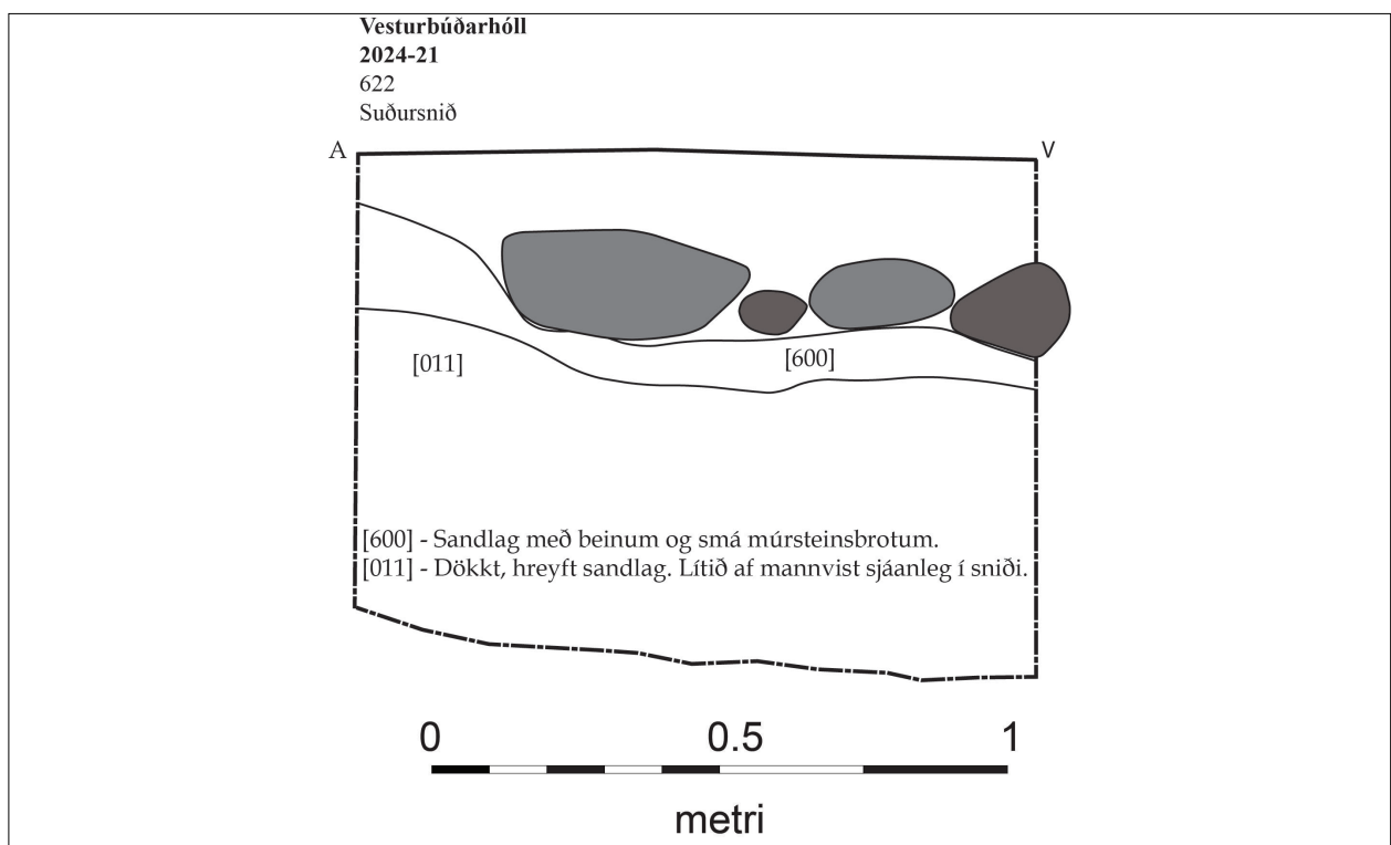
Mynd 14. Teikning af suðursniði könnunarskurðs [622].
