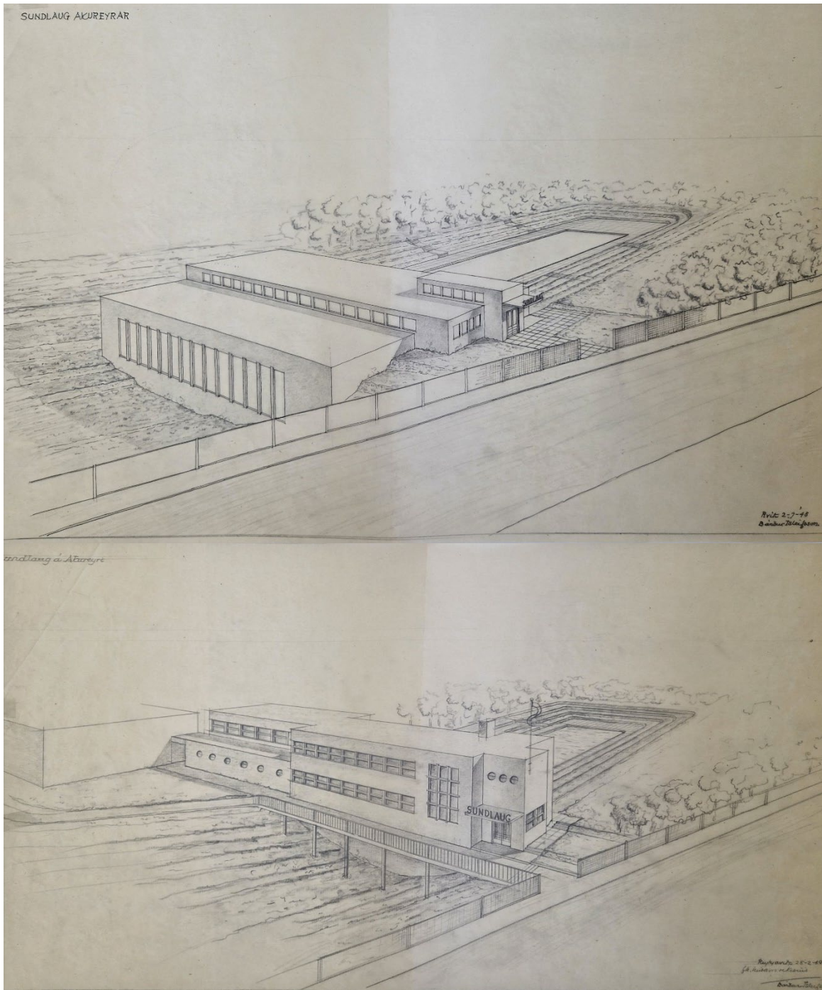
Tvær tillögur að nýrri byggingu sundlaugar Akureyrar. Sú efri er frá 2. júlí 1948 en sú neðri frá 28. febrúar 1949 en báðar eru þær merktar Bárdi Ísleifssyni. (Húsameistari ríkisins, Djóðskjalasafn Íslands C383_07). Á neðri myndinni er húsið farið að líkjast nokkuð endanlegri byggingu þótt viðbygging sunnan við hefði ekki risið heldur innisundlaugin endað í kjallara norðurbyggingar.
