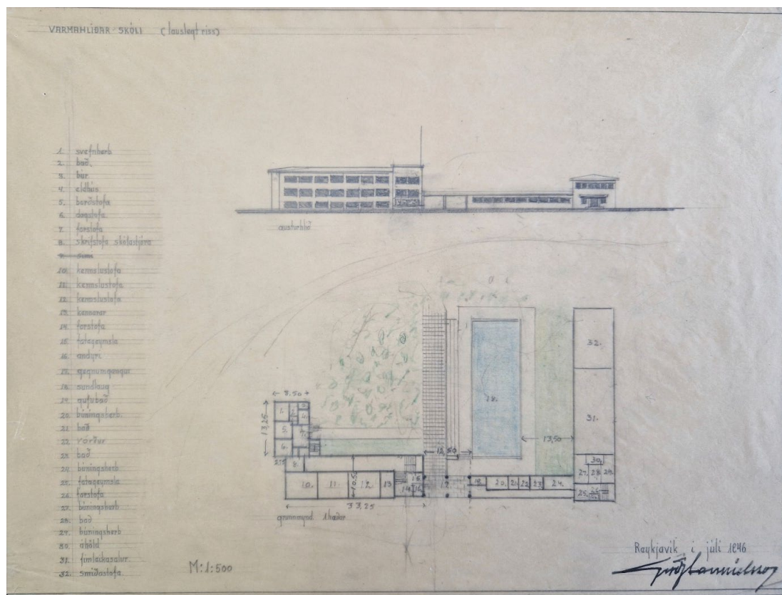
Teikning Guðjóns Samúelssonar að Varmahlíðarskóla dagsett í júlí 1946. (Teikningasafn Húsameistara ríkisins.)
