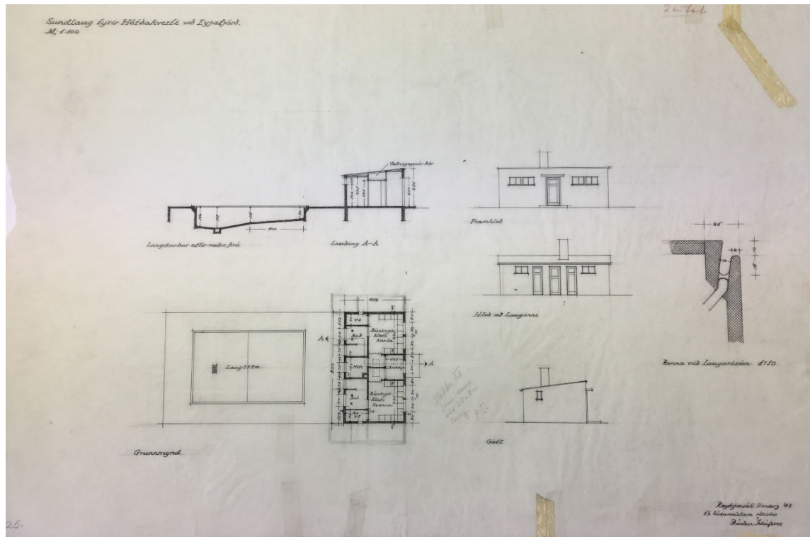
Gljúfralang, Grenivík. Teikningin er merkt Bárði Ísleifssyni/Húsameistara ríkisins 9. mars 1943. Teikning úr safni Íþróttarsjóðs, Þjóðskjalasafn Íslands H26.
