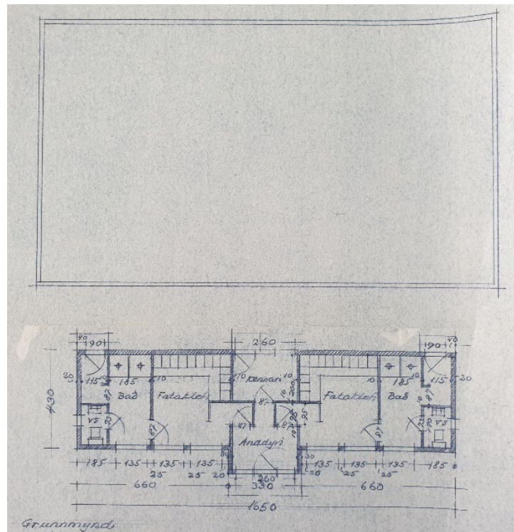
Tillaga Bárðar Ísleifssonar að búningsklefabúsi við Barðslaug, dagsett 1962. Húsið var ekki byggt. Húsameistari ríkisins.
