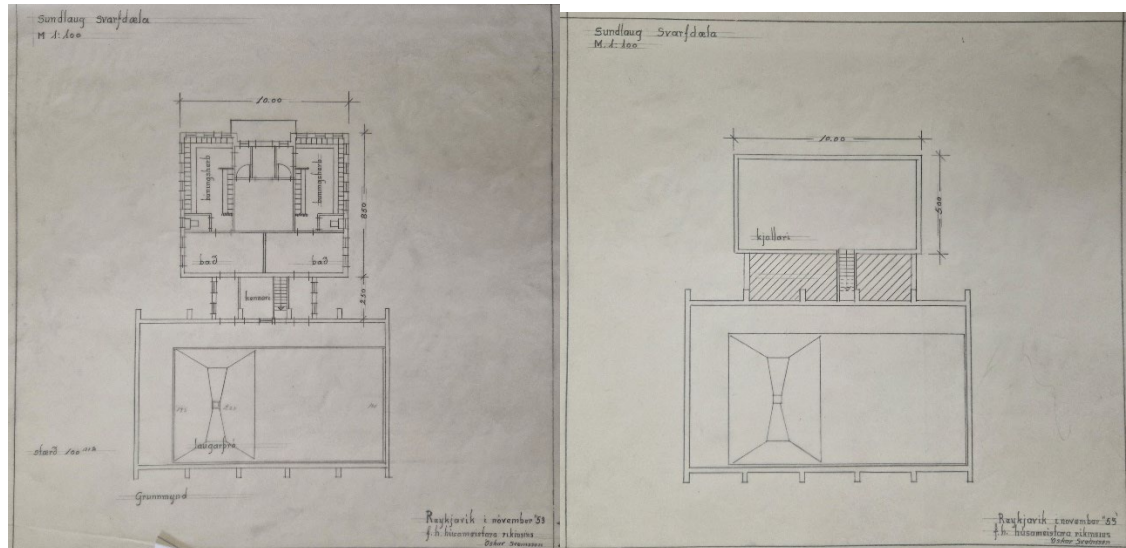
Teikning Óskars Sveinssonar að nýrri bíningsaðstöðu dagsett í nóvember 1953 fyrir bönd Húsameistara ríkisins. Húsameistari ríkisins, C393_07, Þjóðskjalasafn Íslands
