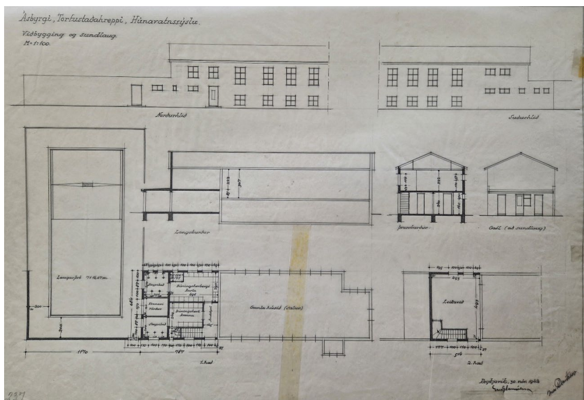
Teikning af sundlaug og bíningsbúsi sem tengdi sundlaug og samkomuheimili. Teikningin er merkt Guðjóni Samúelsyni og frá 30. nóvember 1942 en í hornið kvittar einnig Már Ríkardsson. Varðveitt í gögnum Húsameistara ríkisins, C384-02.
