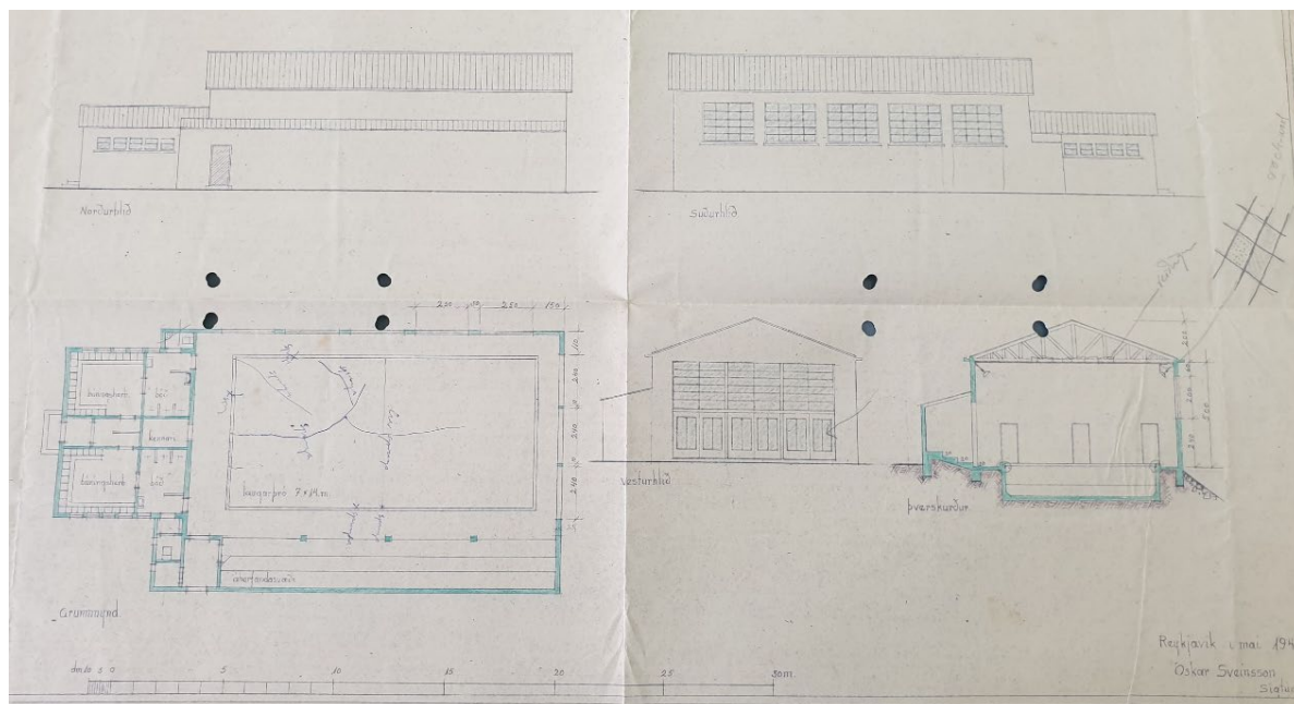
Hugmynd að framkvæmdum við sundlaugarhús á Syðra-Laugalandi frá 1946. Teikningin er merkt Óskari Sveinssyni en hún virðist vera hugmynd að stærkun þess húss, sem þá var á staðnum, en ekki hafa orðið að veruleika. Þjóðskjalasafn, H26 Teikningar Íþróttasjóðs.
