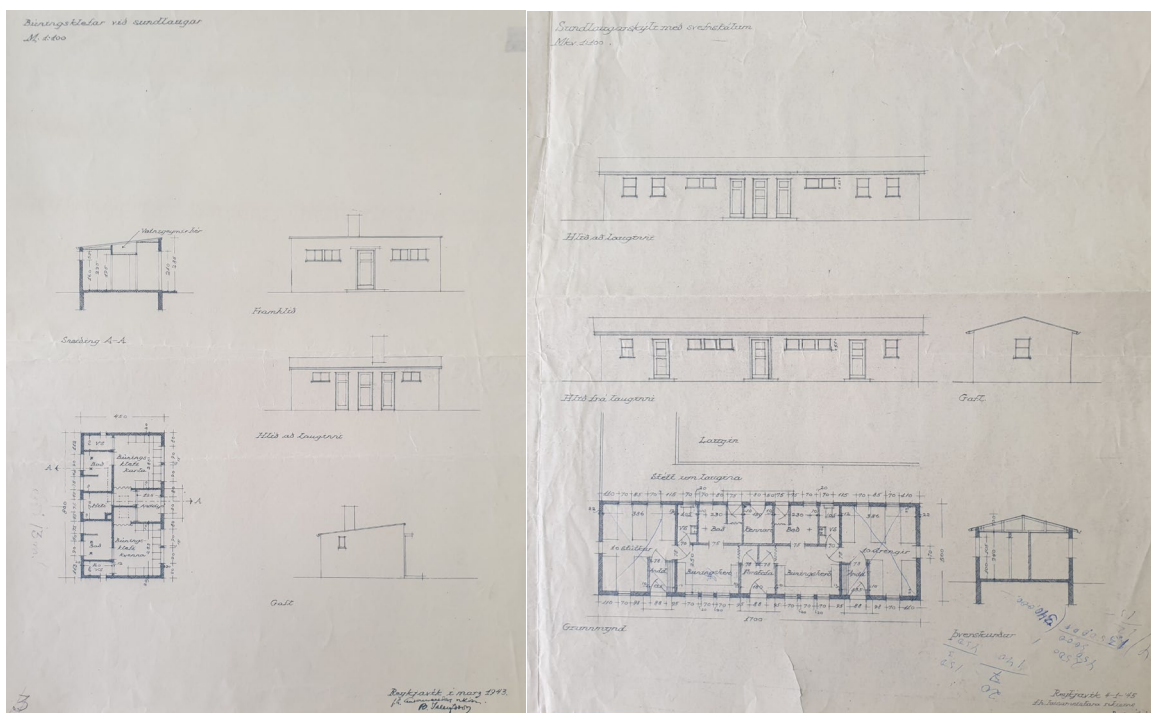
Mynd 10-11: Tvær gerðir af dæmigerðum laugarhúsum frá fyrri hluta 20. aldar. Til vinstri er „sýnidæmi“ um sundlaugarbyggingu sem var að finna með gögnum um gömlu Varmárlaugina, en ekki fannst eiginleg teikning af eldri sundlaugarhúsi þar. Teikningin er merkt Bárði Ísleifssyni/ húsameistaraskrifstofu ríkisins, Reykjavík í mars 1943. Þjóðskjalasafn, H25 Teikningar Íþróttasjóðs. Til hægri er tillaga Húsameistara ríkisins að sundlaugarhúsi og heimavist. Þjóðskjalasafn Íslands H25 – Teikningar Íþróttasjóðs.
