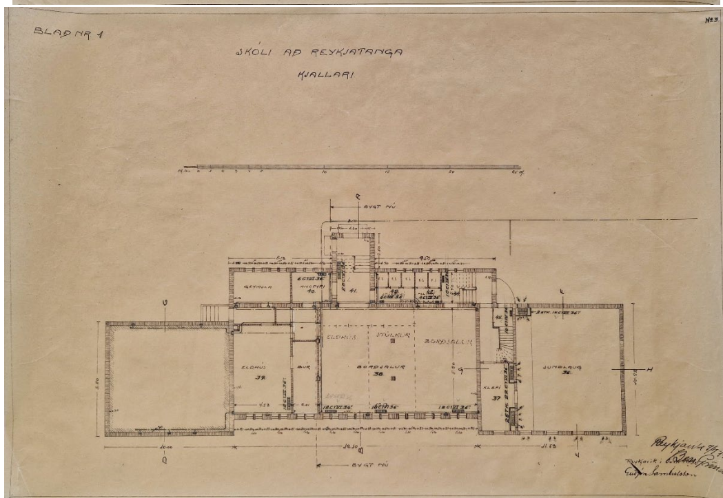
Teikning af býráðsskóla á Reykjanesi frá september 1930, undirrituð af Guðjóni Samúelssyni en yfirstrikað og merkt Ben Gröndal. Húsameistari ríkisins, C0999_01.
