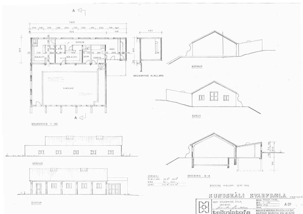
Teikning Hauks Haraldssonar dagsett í ágúst 1986 að nýjum búnings- og baðklefum við vesturblið Sundskálans. Dalvíkurbyggð.is, kortavefur.
