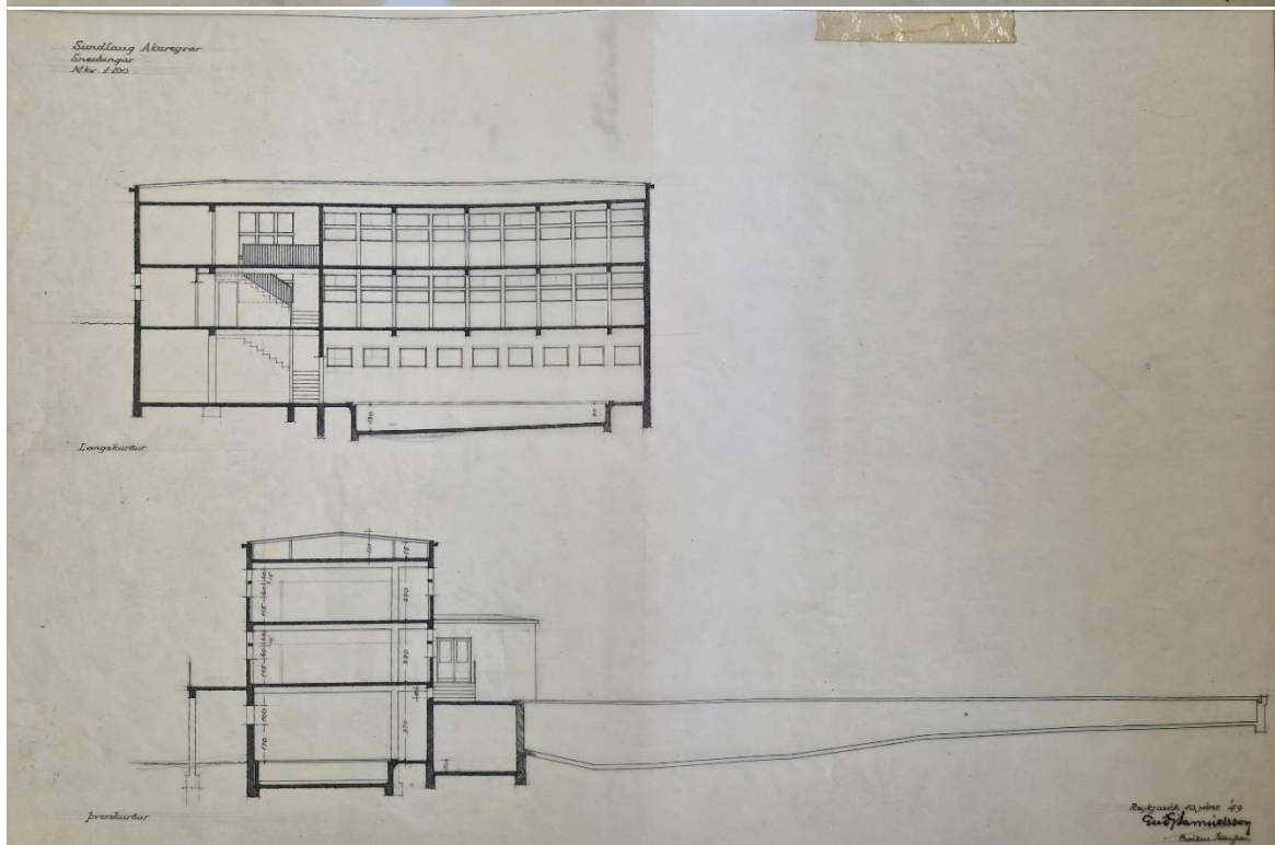
Sundlaug Akureyrar á teikningum frá 1949. Teikningar eru merktar Guðjóni Samúelsyni/ Bárði Ísleifssyni Húsameistari ríkisins C383_07, Þjóðskjalasafn Íslands.
