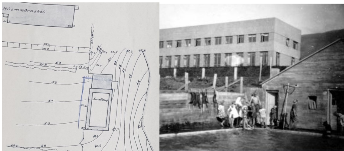
Stærð og staðsetning laugar og laugarhúsa frá 1934. Til vinstri er lausleg uppmæling frá Verkefræðistofu Sigurðar Thoroddsen sem varðveitt er á meðal gagna Íþróttasjóðs (H26, Þjóðskjalasafn Íslands). Á ljósmyndinni má sjá bluta af húsinu lengst til hægri á mynd. Mynd úr Sarpi STÆ1-6998.
