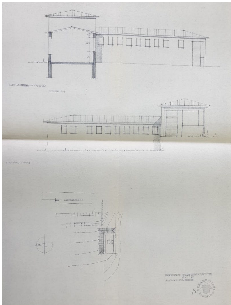
Teikning af nýja laugarhúsinu sem byggt var 1964 eftir að eldra hús hafði verið rífið. Arkitekt: Guðmundur Guðjónsson/Húsasmiðameistari ríkisins. Þjóðskjalasafn, H26 Teikningar Íþróttasjóðs.
