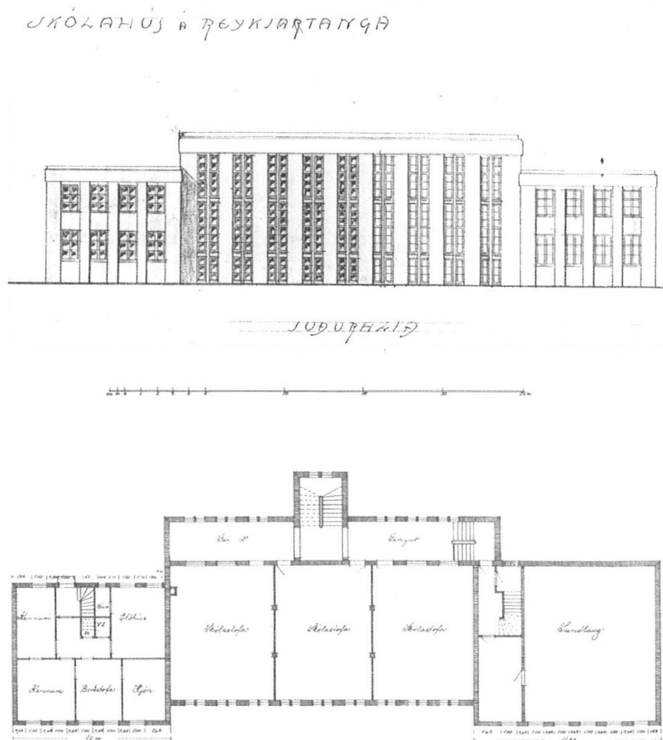
Skólabús og sundlaug að Reykjum í Hrílafirði. Að ofan eru frumdrög að suðurhlíð húss frá júní 1930 og að neðan innri skipan. Teikningar úr bók Péturs Ármannssonar. 2020, bls. 200.
