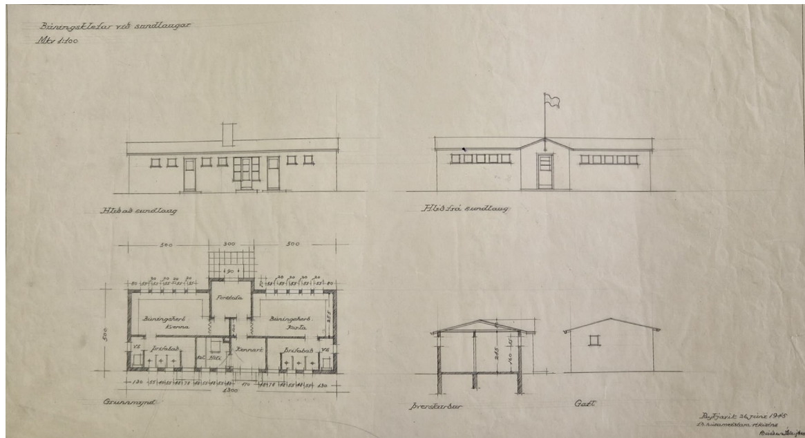
Stöðluð laugarteikning Bárðar Ísleifssonar frá júní 1945 sem laugarhús á Þelamörk virðast byggð eftir. Húsameistari ríkisins C388_09-10. Gögn Húsameistarar ríkisins, Þjóðskjalasafn Íslands.
