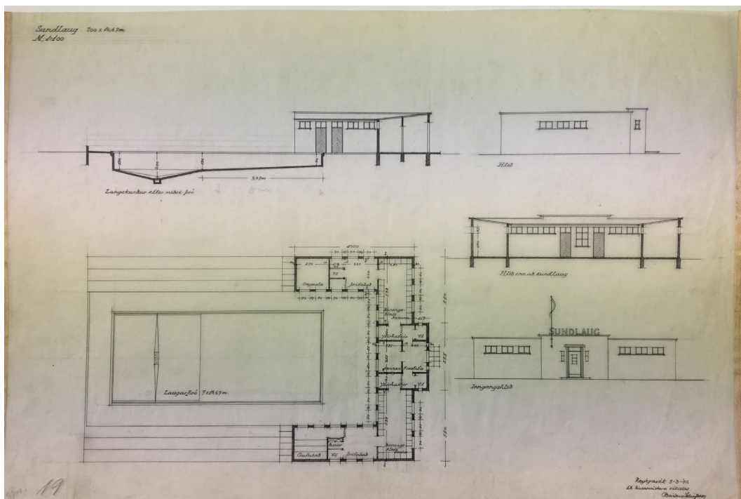
Mynd 12: Teikning af sundlauginni á Þórshöfn, dagsett 5. mars 1942 og undirrituð af Bárði Ísleifssyni fyrir hönd Húsameistara ríkisins. Varðveitt á Þjóðskjalasafni Íslands. Laugin á Þórshöfn var nýlega rífin.
