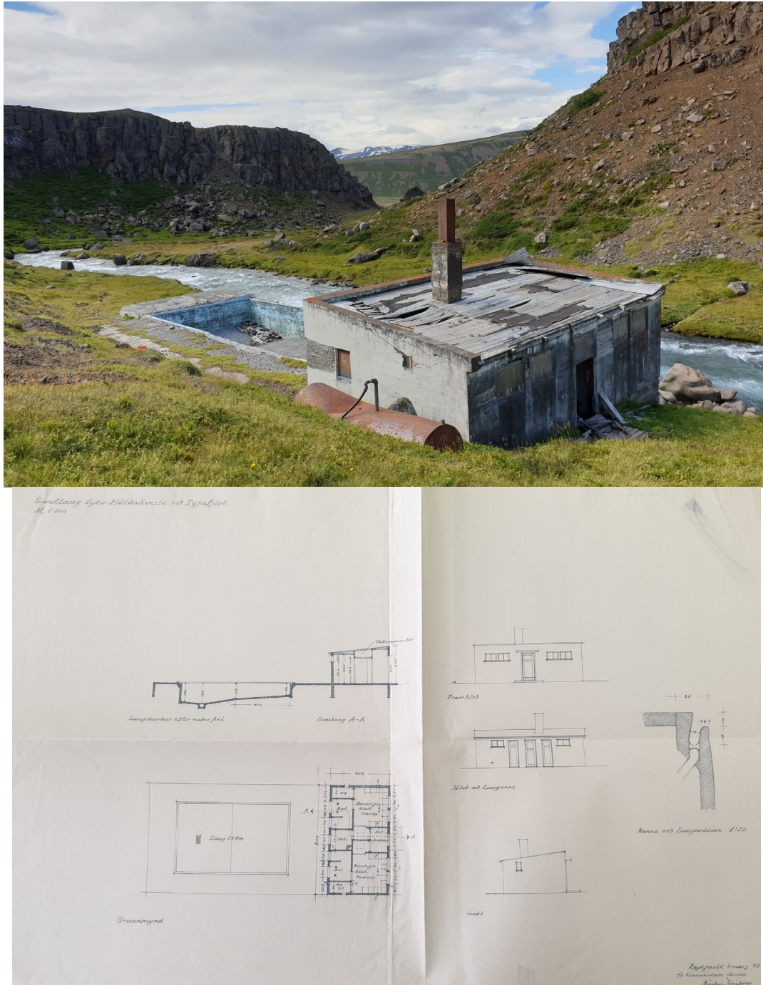
Mynd 5: Teikning af Gljúfrlaug í Gýtubakkahreppi, dagsett 9. mars 1943, undirrituð af Bárði Ísleifssyni, fyrir hönd Húsameistara ríkisins (neðar). Teikningin er varðveitt á Þjóðskjalasafni Íslands. Sundlaugin var byggð af slýsavarnafélaginu Ægi og sá það um rekstur hennar fyrstu árin. Þegar komið var fram á 9. áratuginn var viðhaldi mjög ábótavant og laugin þótti orðin bæði óhentug og hattuleg. Árið 1988 var því síðasta sumarið sem laugin var opin, en ný sundlaug á Grenivík var opnuð tveimur árum síðar. Sundlaugin er á meðal þeirra lauga sem heimsóttar voru sumarið 2024. Efri mynd: ljósmynd af lauginni: Höfundar.
