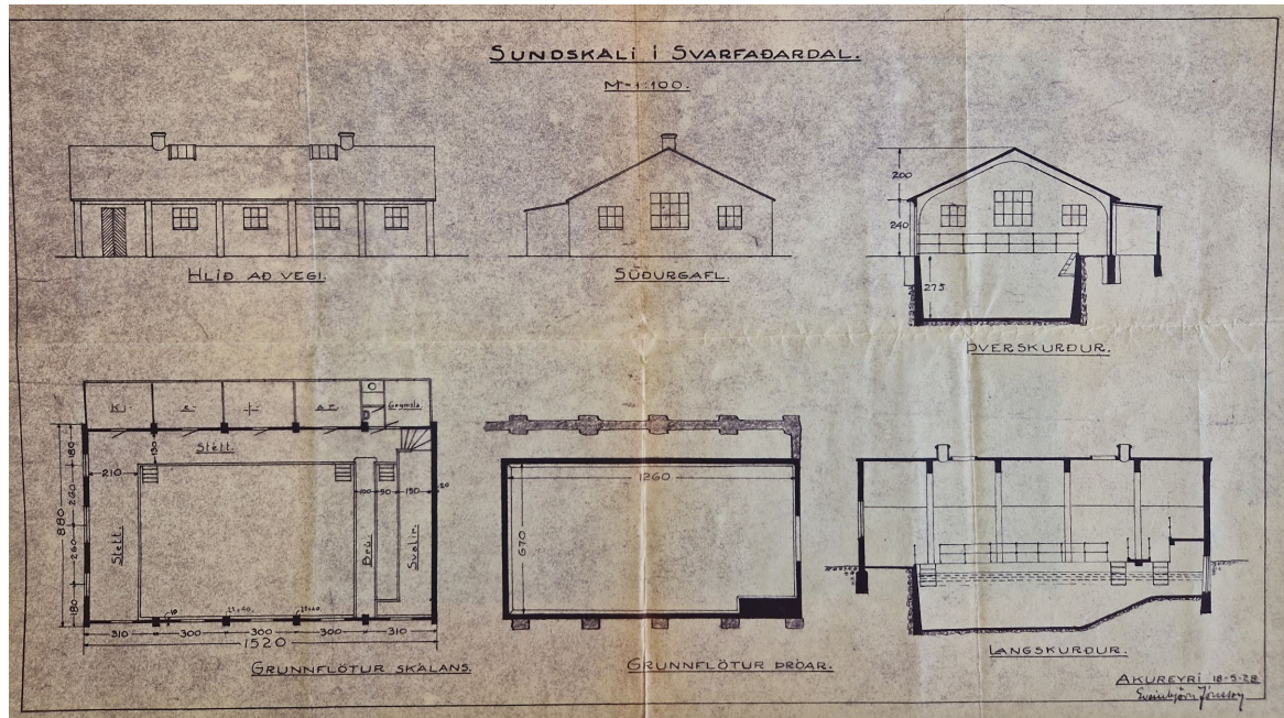
Þriðja teikning Sveinbjarnar, dagsett á Akureyri 18.5. 1928. Teikningasafn Þjóðskjalasafns Íslands 22-6. Einnig Héraðsskjalasafnið á Dalvík.
