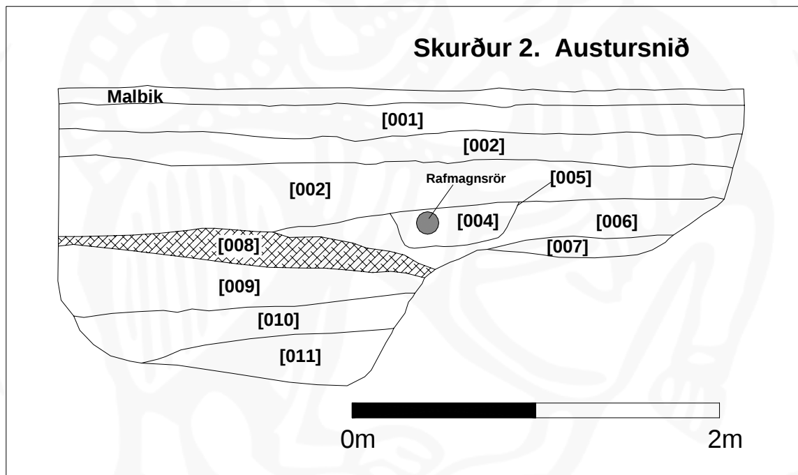
Mynd 4: Teikning af austursniði skurðar 2.
