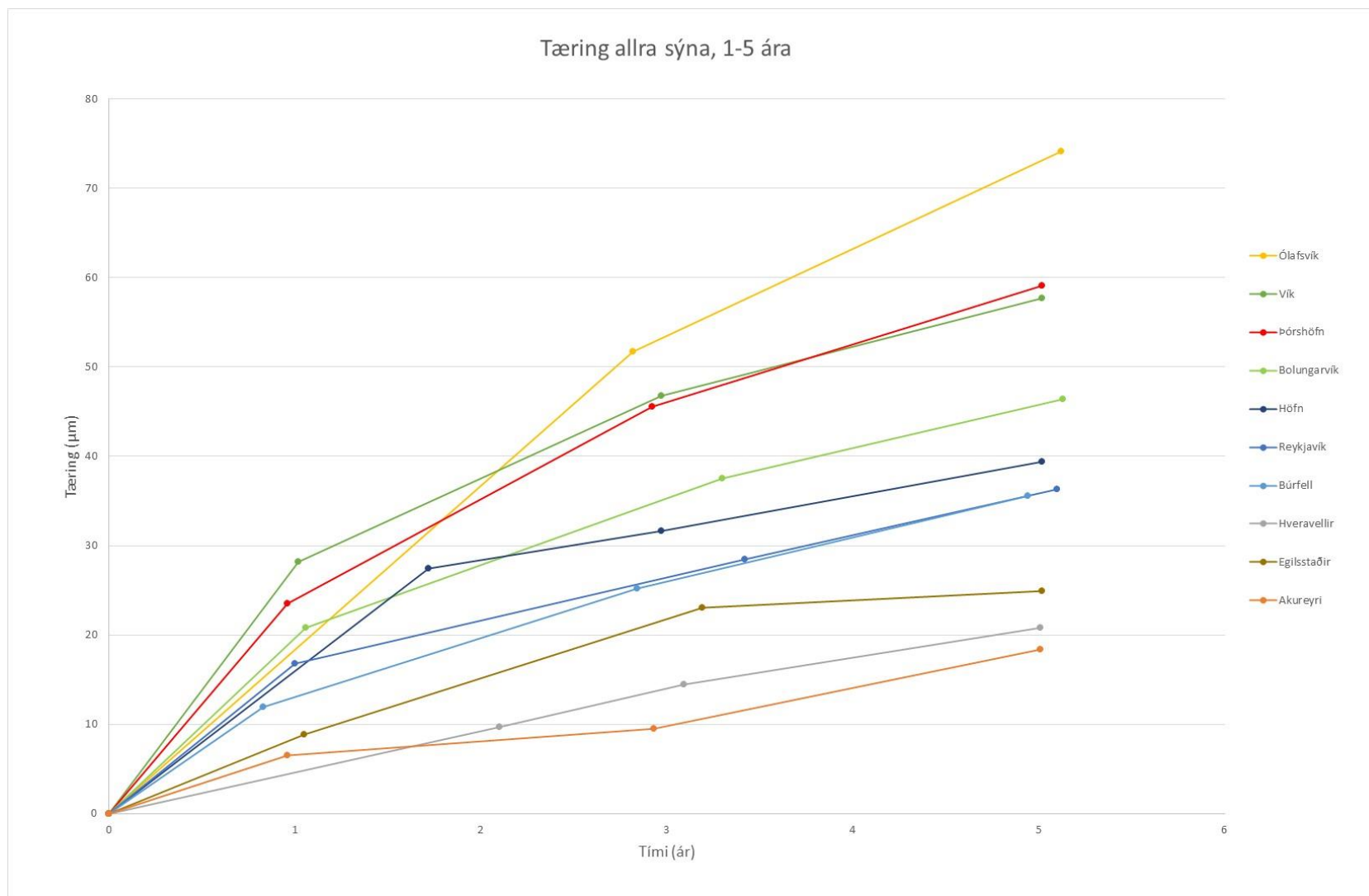
MYND 11 Tæring allra sýna sem mæld hafa verið, 1-5 ár.
