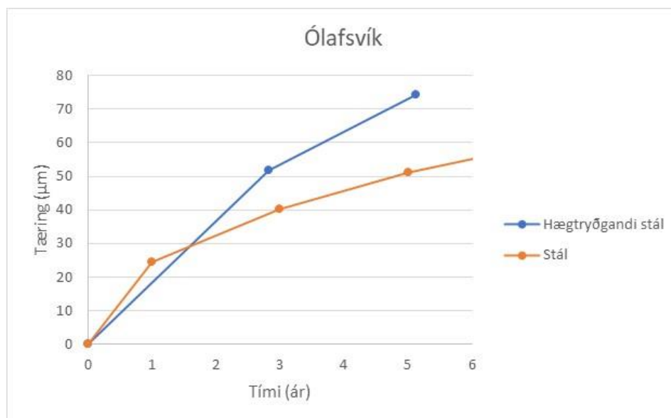
MYND 2 Samanburður á hægtryðgandi stáli og stáli í Ólafsvík eftir 5 ára mælingar.
