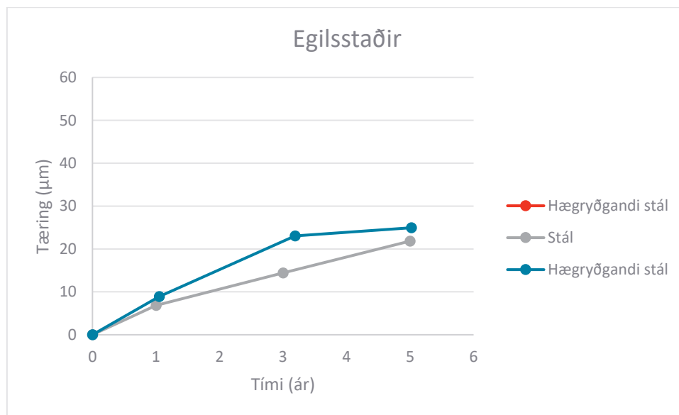
MYND 4 Samanburður á hægryðgandi stáli og stáli á Egilsstöðum eftir 5 ára mælingar.
