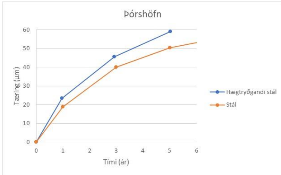
MYND 7 Samanburður á hægtryðgandi stáli og stáli á Þórshöfn eftir 5 ára mælingar.
