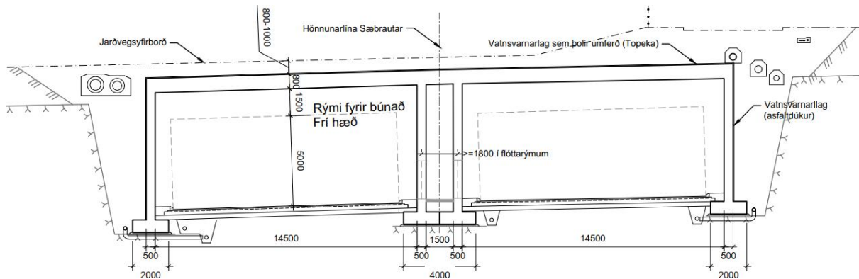
Mynd 4.3 Dæmigert þversnið í steypnan stökk samkvæmt frumdrögum hönnunar.
