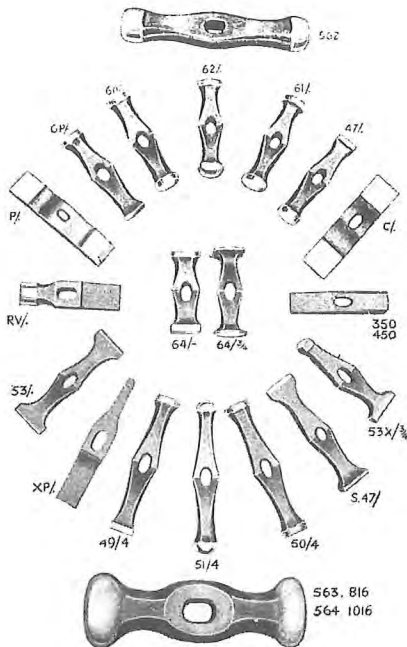
Ýmsar gerðir hamarshausa, sem notaðir eru við blikksmiði.
