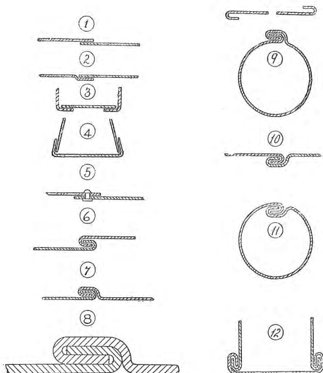
Sýnishorn af lásasamsetningum
