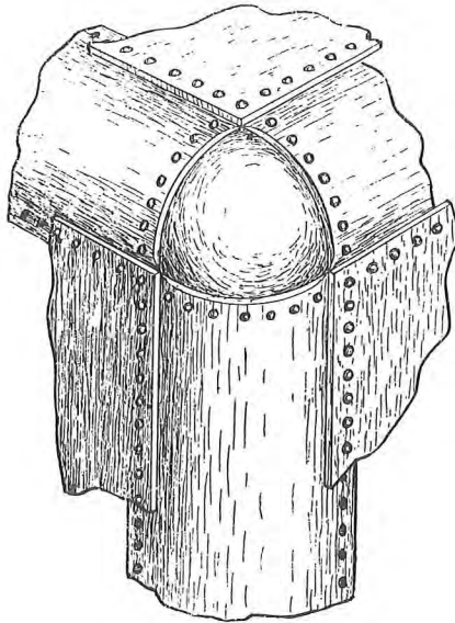
Sýnishorn af samsetningu með slaghnoðum
