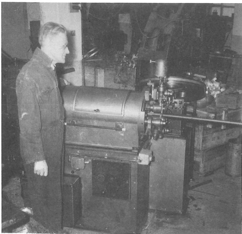
Úr Blikksmiðjunni Gretti. Myndin sýnir eina af hinum flóknu vélum sem þúsundþjalasmiðurinn Karl Stefánsson, (bróðir Ingibergs í Gretti) smíðaði. Í vélinni eru framleidd rör í hitara fyrir lofthitun.
