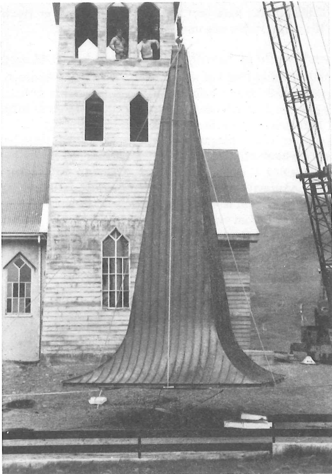
Turnspíra Grundarfjarðarkirkju. Klædd með eir hjá Blikksmiðjunni h.f.
