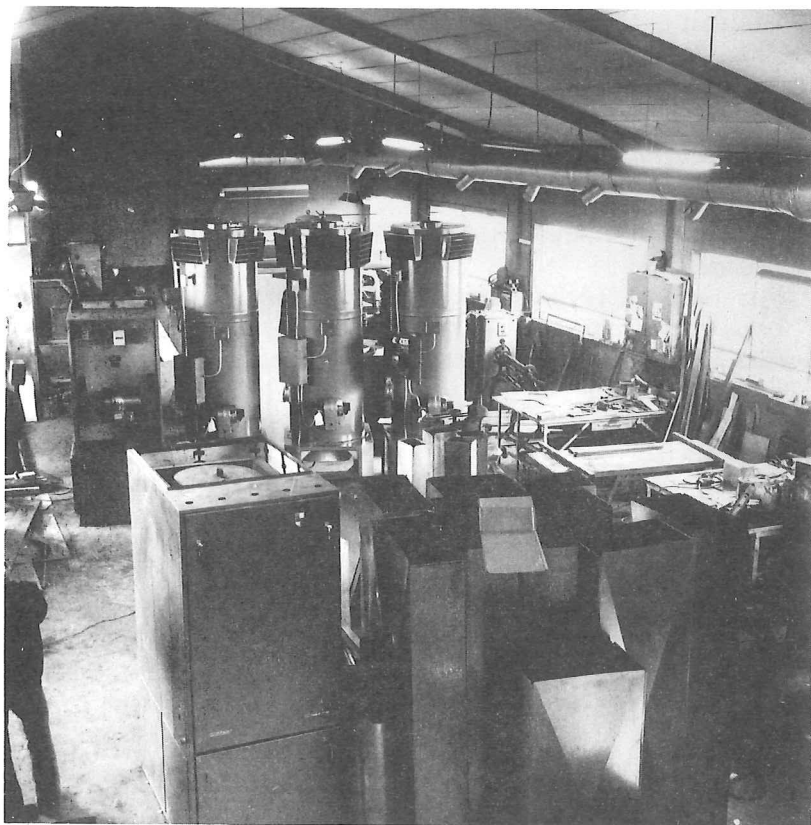
Mynd úr vinnusal Blikksmiðjunnar Glófaxa. Á myndinni má sjá 2 gerðir af loft-hitunarkötlum, þeim er fyrirtækið framleiddi.
