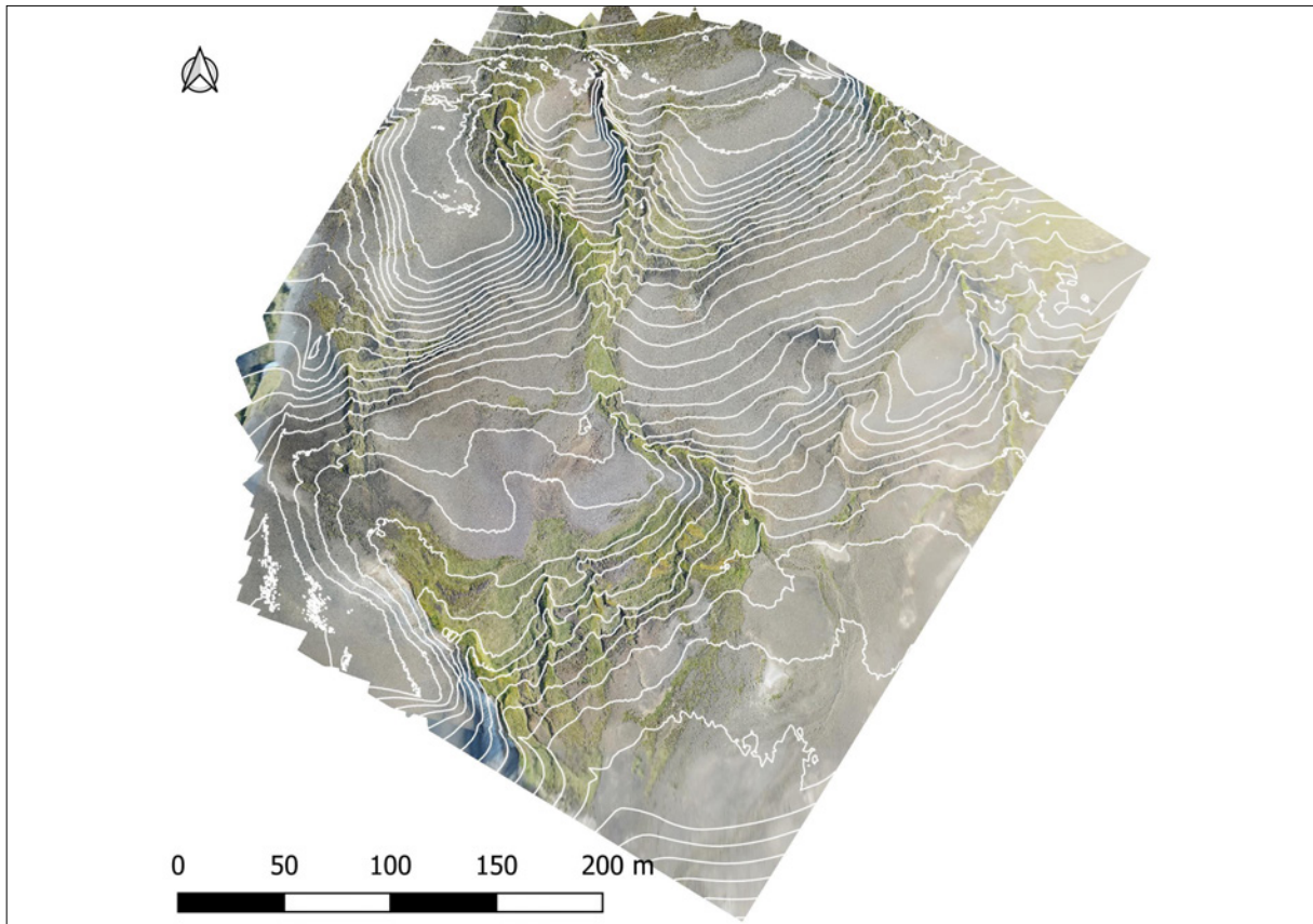
Mynd 4. Undir Lambhöfða. Hnitúð, samsett loftmynd (OP) með 1 m hæðalínunum.
