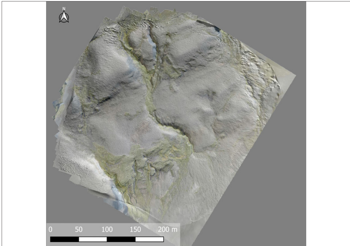
Mynd 6. Undir Lambhöfða. Hæðaskuggar (hillshade) með 50% gegnsæi yfir hnitaðri, samsettri loftmynd. Hér sést vel móta fyrir skála og fjósi.
