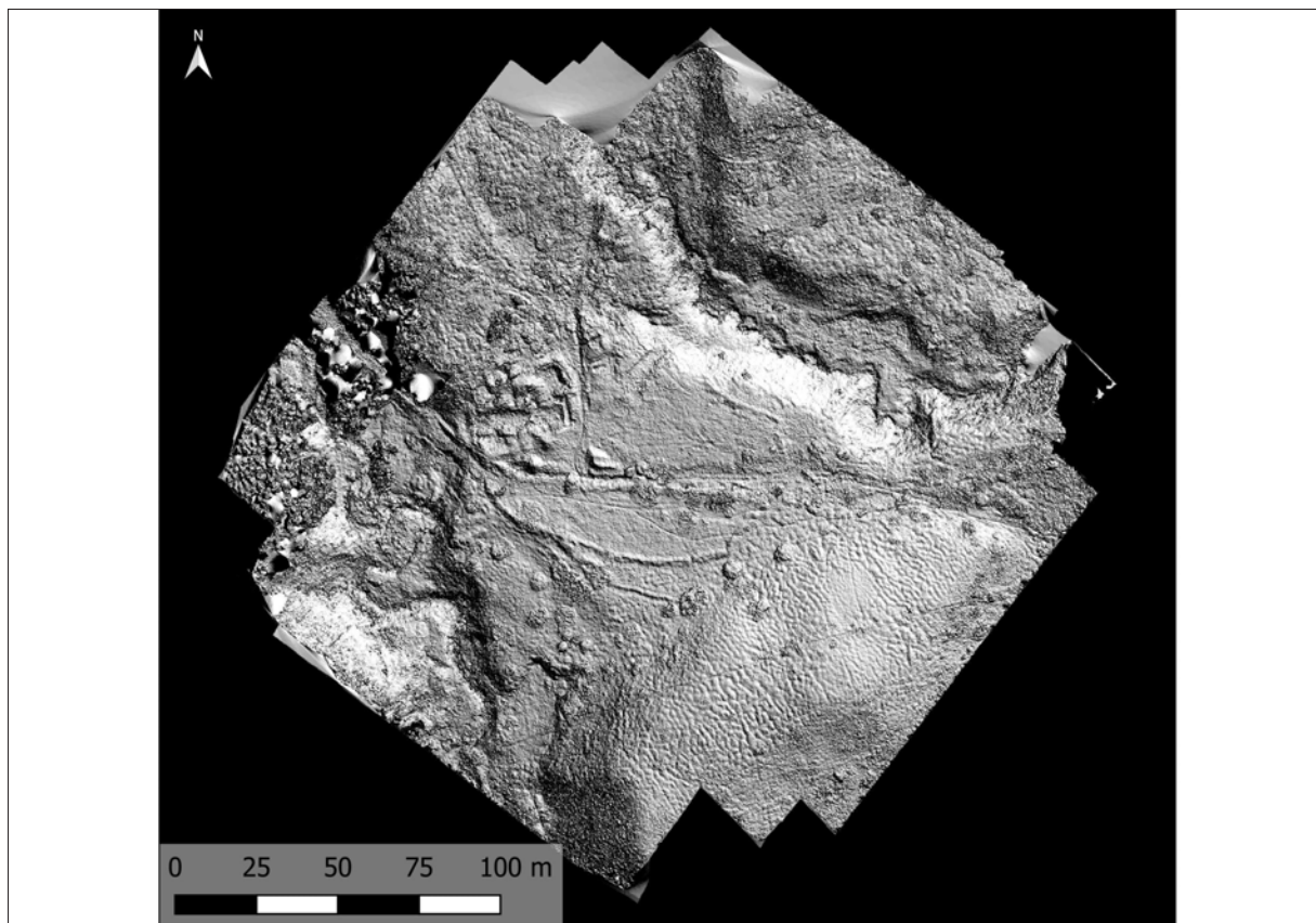
Mynd 9. Skallakot. Hæðaskuggar (hillshade). Hér sést einnig móta vel fyrir minjum og uppgraftarsvæði.
