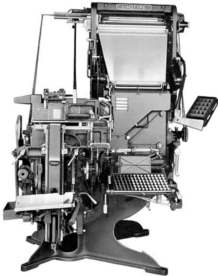
Setjarinn sat við lyklaborðið t.h. og skráði textann. Vélin raðaði stafamótum í línulengd. Línurnar steypar í blý og komu á bakkann t.v.
