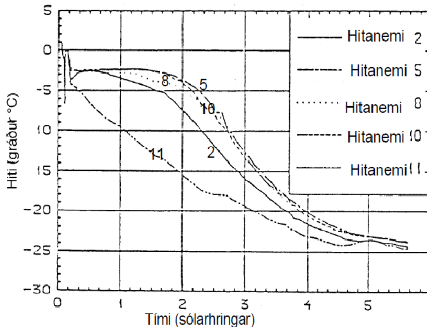
Mynd 1. Hitapróun í fiskblökkum sem er staflað á bretti og settar hálfrosnar í frystilest. Hitanemum er komið fyrir á mismunandi stöðum í fiskblökkum á bretti (Magnussen, 1988).
