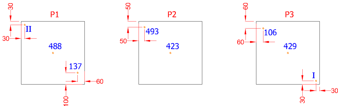
Mynd 4. Grunmynd af staðsetningum hitasírta innan í grálúðupokum. Sírtar eru táknaðir með appelsínugulum punkti og númer þeirra er í bláum lit. Málsetningar eru í millimetrum (mm) og var sírtum komið fyrir í miðri hæð hvers poka.
