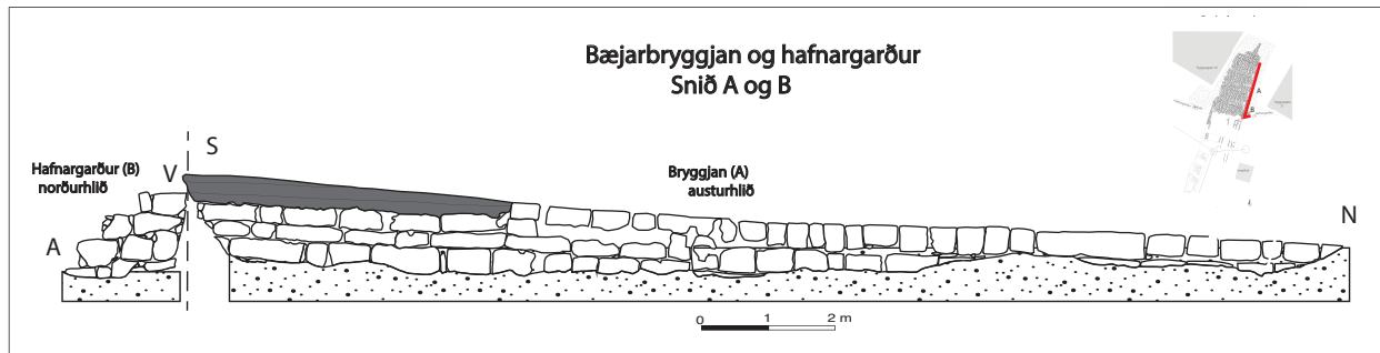
10 Austursnið Steinbryggju og hafnargarður frá 1928. Innfellda myndir sýnir staðsetningu sniðanna
