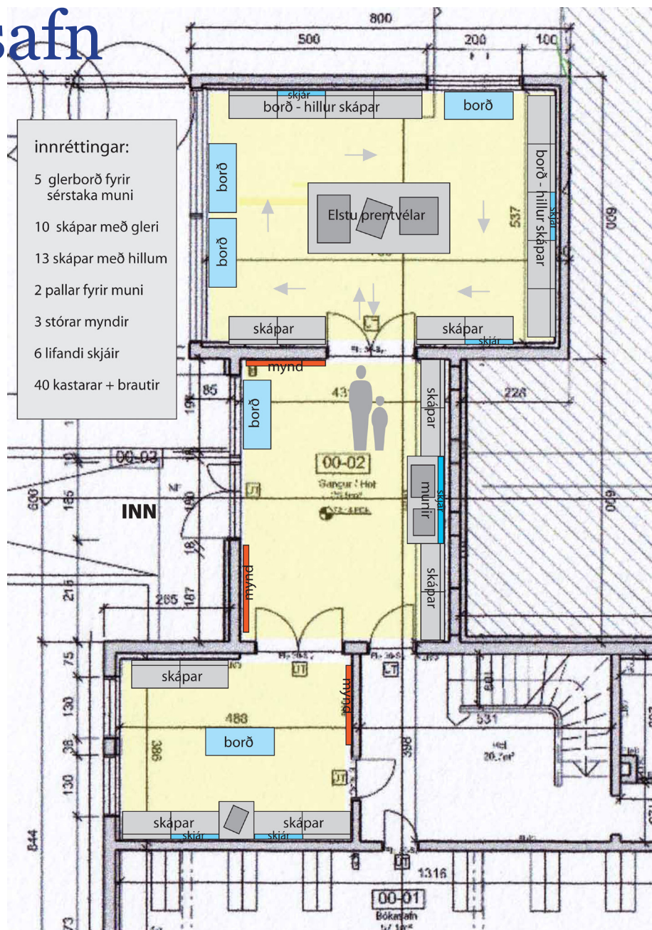
SKÁLHOLT - GESTAHÚS - PRENTSÖGUSETUR Í KJALLARA Mkv. 1:50
