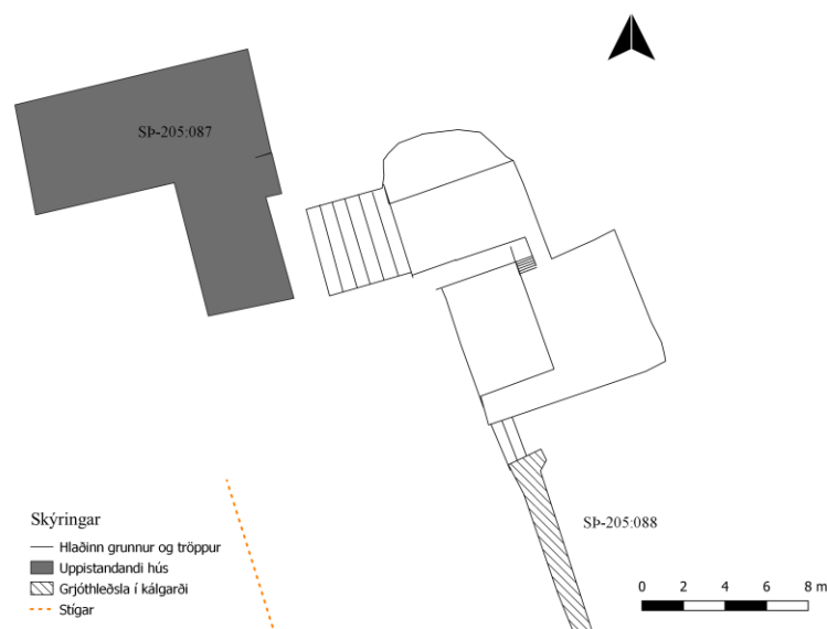
Uppmæling á þeim ummerkjum sem enn sjást um hús Bárðar Sigurðssonar, Sp-205:047
