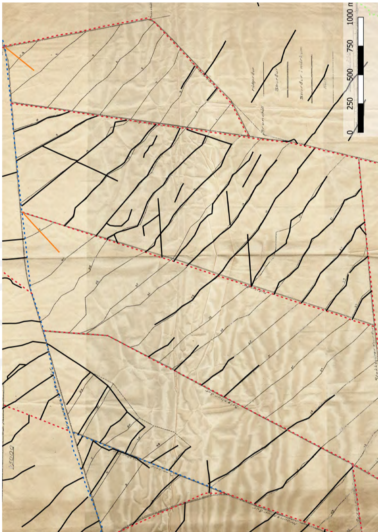
Á myndinni er áveitukort Stokkseyrarhverfis. Svartar línur eru flóðgarðar, bláar línur aðfærslukurðir, appelsínugular línur innrásir og rauðar línur þurrrskurðir. Hér sést vel hvernig hönnun og raunveruleika ber ekki saman, á kortinu er fjöldi flóðgarða sýndur sem aldrei voru hlaðnir. ©Héraðsskjalasafn Árnesinga og Fornleifastofnun Íslands.
