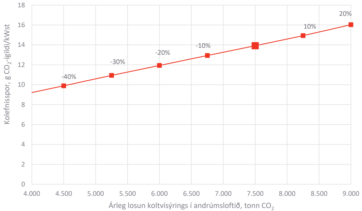
MYND 25 Næmnigreining á kolefnisspori vegna vinnslu á 1 kWst í þeistareykjastöð (án raforkuflutnings) með breytilegri beinni losun koltvísýrings (CO 2 ) í andrúmsloftið.
