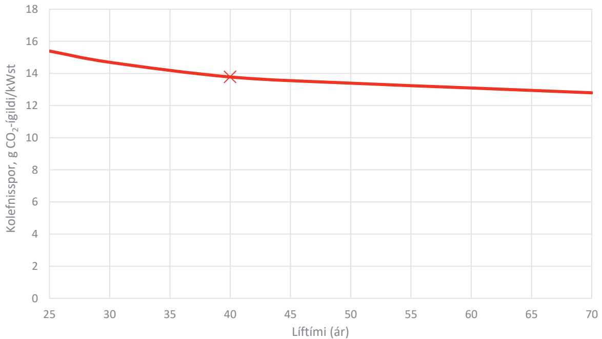
MYND 24 Næmnigreining á kolefnisspori vegna vinnslu á 1 kWst í Þeistareykjastöð (án raforkuflutnings) með breytilegum líftíma.
