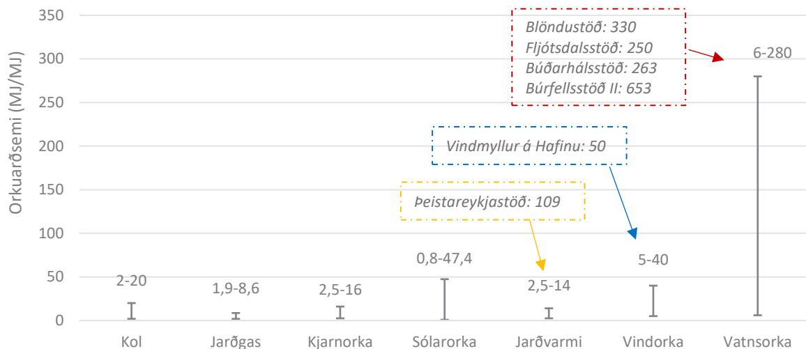
MYND 22 Birtar niðurstöður fyrir orkuarðsemi mismunandi orkugjafa [2, 3, 27, 5, 4, 6].
