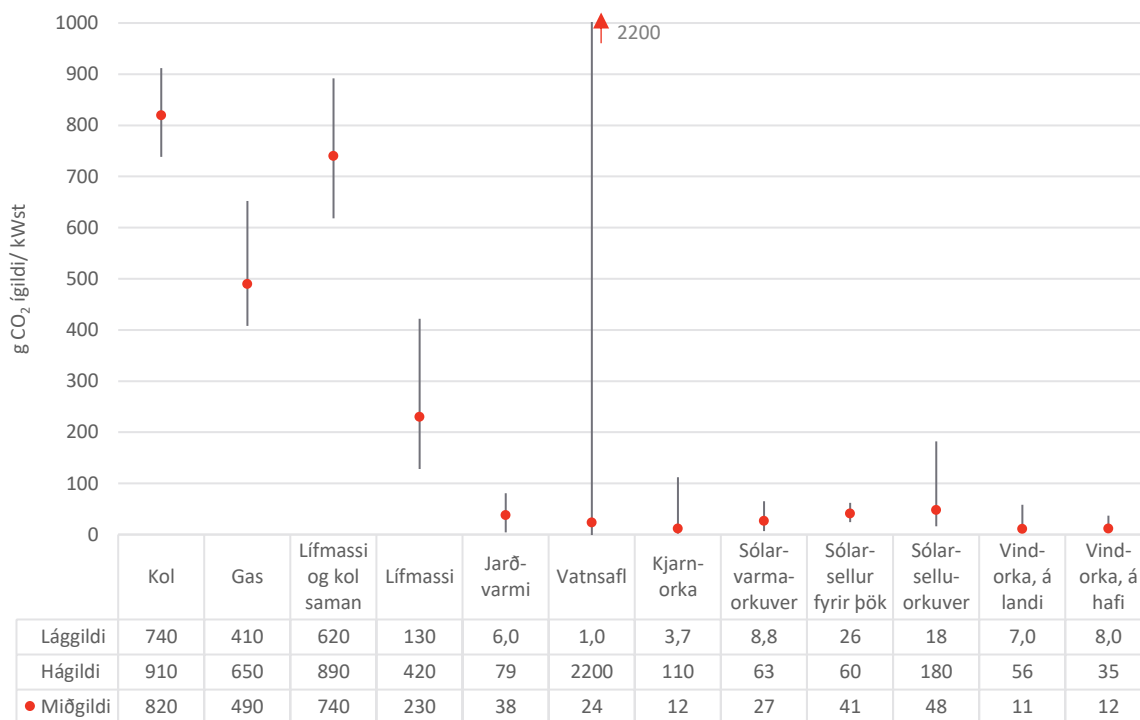
MYND 30 Losun gróðurhúsalofttegunda frá vinnslu raforku með mismunandi orkugjöfum í g CO 2 ígilda fyrir unna kWst. Myndin byggir á samantekt IPCC frá árinu 2014 [47] og sýnir miðgildi (rauður punktur), há- og lággildi frá niðurstöðum vistferilsgreininga fyrir hvern orkugjafa. Frá því að þessi samantekt var gefin út hafa verið birtar niðurstöður fyrir jarðvarma með losun allt að 1.800 g CO 2 -ígildi/kWst. Kolefnisspor Þeistareykjavirkjunar er 13,8 g CO 2 ígildi/kWst án raforkuflutnings.
