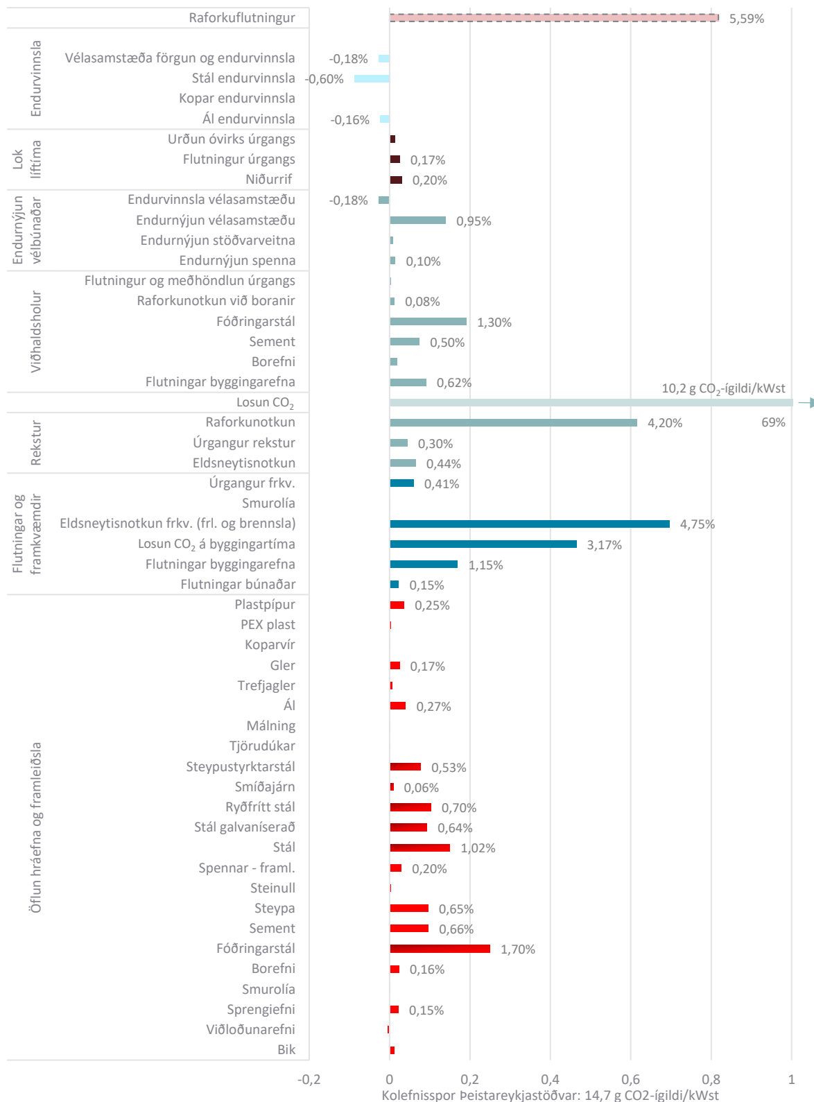
MYND 20 Gróðurhúsaáhrif einstakra þátta í kolefnisspori þeistareykjastöðvar. Athugið að x-ás stoppar við 1 g CO 2 -ígildi/kWst, en bein CO 2 losun er mun hærri eða 10,2 g CO 2 -ígildi/kWst.
