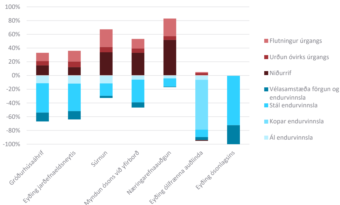
MYND 17 Hlutdeild ólíkra rekstrarþátta fyrir hvern flokk umhverfisáhrifa, vegna vinnslu 1 kWst raforku í Þeistareykjastöð. Á myndinni má sjá niðurstöður fyrir þá sjö flokka umhverfisáhrifa sem reiknað er fyrir á 40 ára líftíma.
