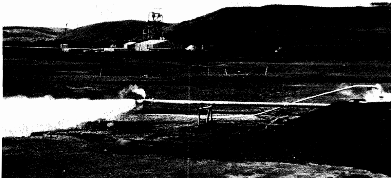
Lokið var á árinu 1966 tæknilegum undirbúningi að gufuveitu til Kísilgúrverksmiðjunnar við Mývatn. Hér sést ein af borholum ríkisins í Bjarnarflagi við Námafjall. Í baksýn er Kísilgúrverksmiðjan í byggingu.
