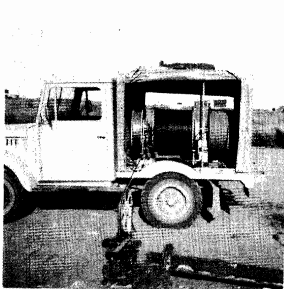
Mælingabíll jarðhitadeildar hefur stórbætt aðstöðu til rannsókna á borholum.
