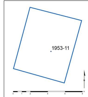
Mynd 31. Teikning af ummáli braggagrunns (1953-10), eftir uppmælingu.
