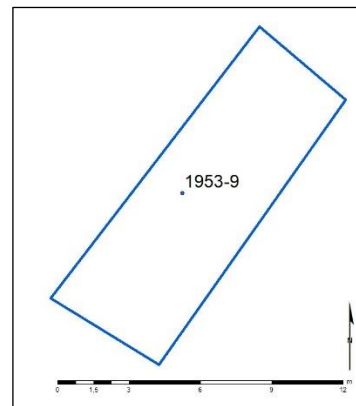
Mynd 27. Teikning af ummáli braggagrunns (1953-9), eftir uppmælingu.
