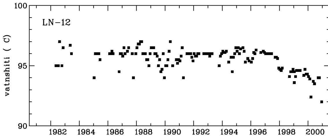
Mynd 8. Hiti vatns úr holu LN-12 á Syðra-Laugalandi árin 1982 - 2000.
