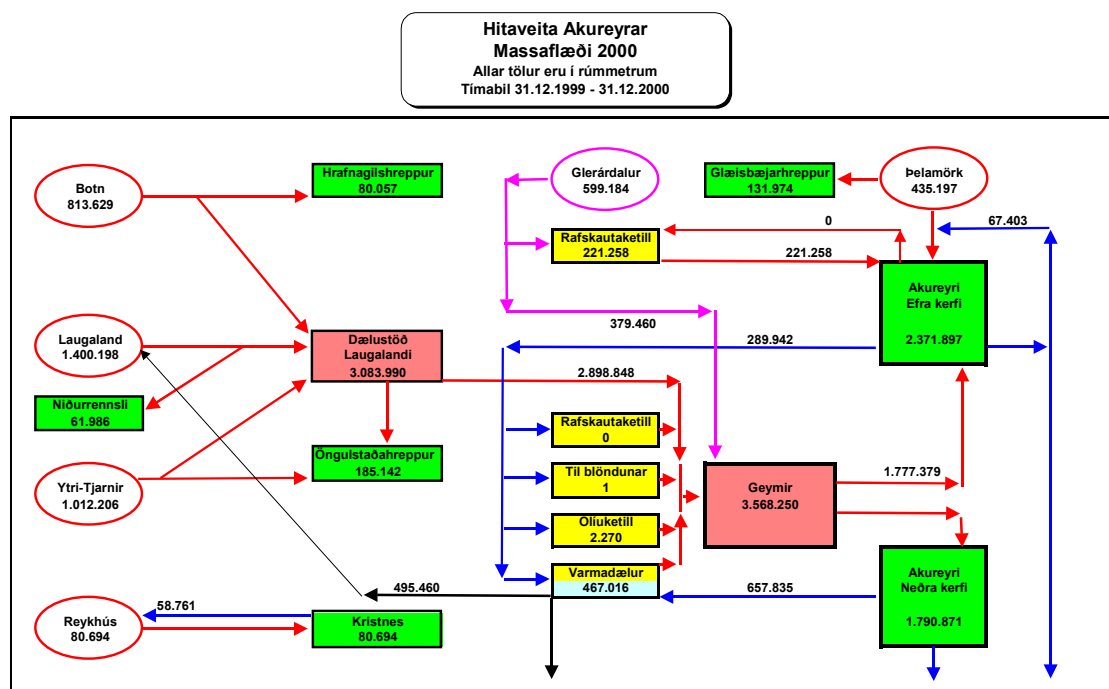
Mynd 12. Heildarorkuflæði um dreifikerfi Norðurorku árið 2000. Tölurnar sýna orkuna sem unnin var úr jarðhitasvæðunum og þá sem framleidd var með öðrum hætti og hvernig hún dreifðist um kerfið.
