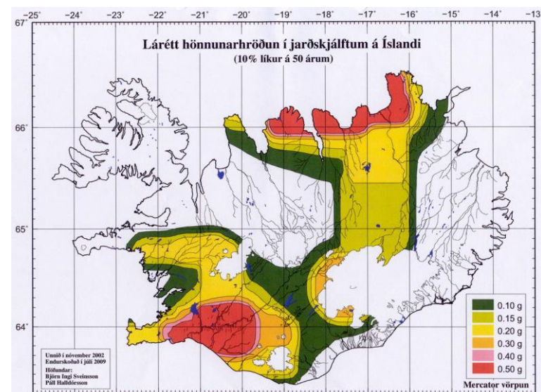
Mynd 5.15. Skipting Íslands í hönnunarhröðunarsvæði miðað við 500 ára meðalendurkomutíma.
