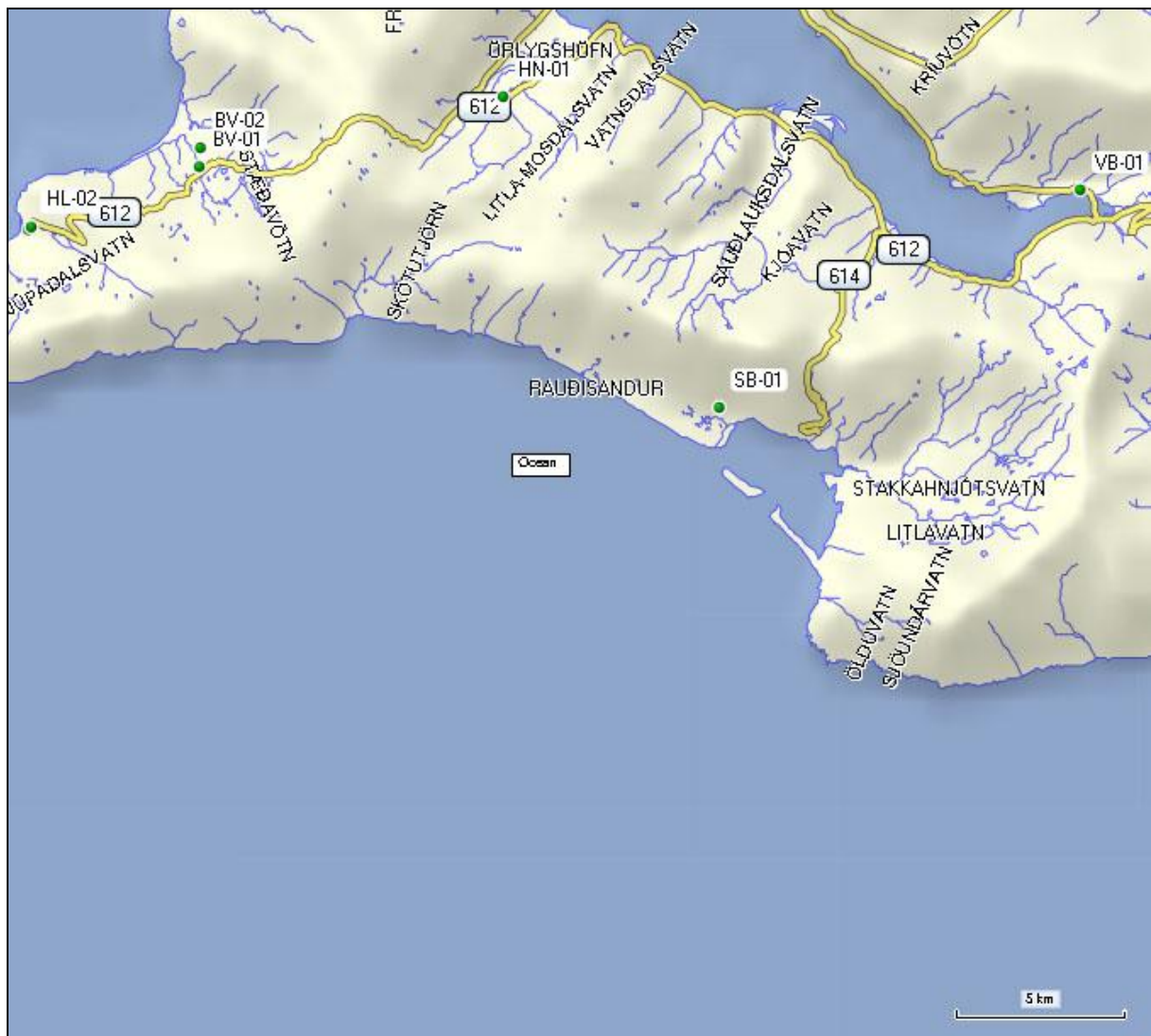
1. mynd. Staðsetning borholna í Rauðasandshreppi.
