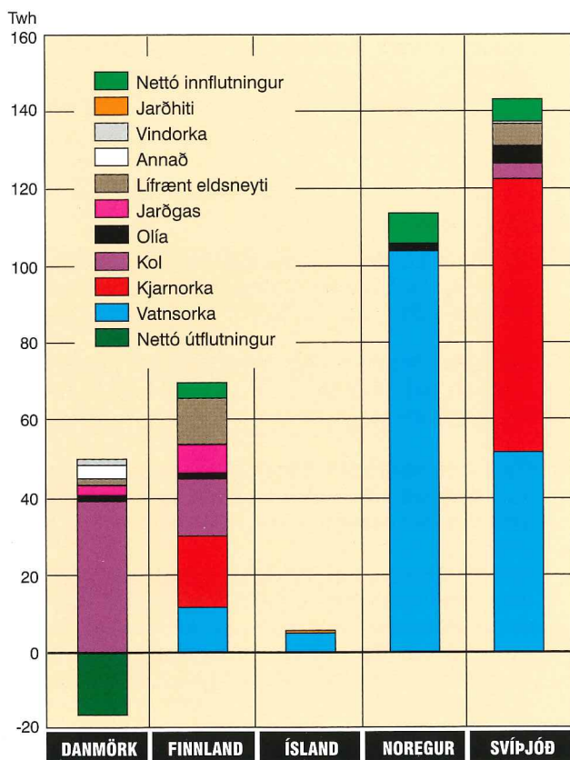
Vinnsla, inn- og útflutningur á raforku á Norðurlöndunum árið 1996. Heimild: Ársskýrsla Nordel 1996.
