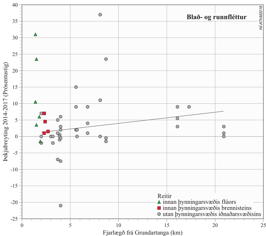
1. mynd. Tengsl fjarlægðar frá Grundartanga (X-ás) og þekjubreytinga (Y-ás) blað- og runnfléttna 2014–2017. Aðhvarfslínan á við um reiti utan þýnningarsvæðisins.
