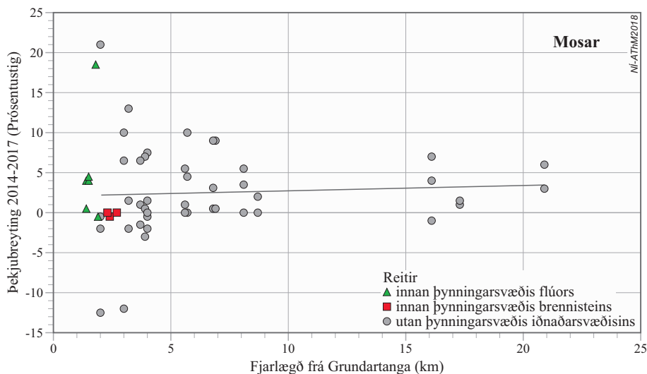
2. mynd. Tengsl fjarlægðar frá Grundartanga (X-ás) og þekjubreytinga (Y-ás) mosa 2014–2017. Aðhvarfslínan á við um reiti utan þýnningarsvæðisins.
