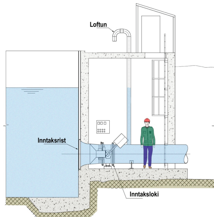
Mynd 5-2 Inntaksmannvirki
