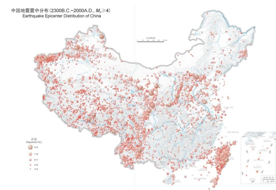
Mynd 10. Skjálftaupptök helstu jarðskjálfta, stærri en M 4 sem hafa orðið í Kína síðustu 4300 árin.
