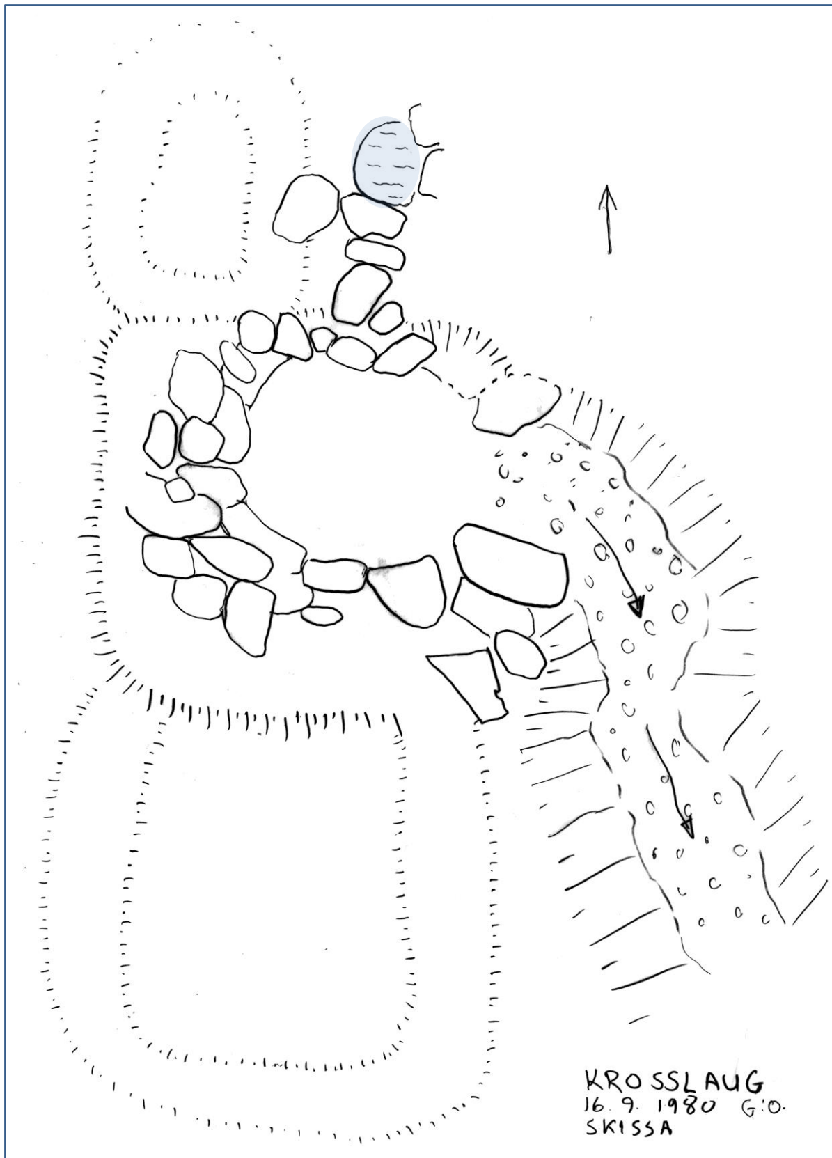
Mynd 3. Skissa af Krosslaug á meðan viðgerð stóð. Leifar af steinhleðslu eru umhverfis laugina og úr suðaustur enda hennar hafði verið grafin rás. Ofan við laugina var lítil uppspretta sem vatn seytleði úr. Hugsanlega vottaði fyrir óljósum minjum bæði sunnan og norðan við laugina (Krosslaug 1980 T-1, G.Ó.).
