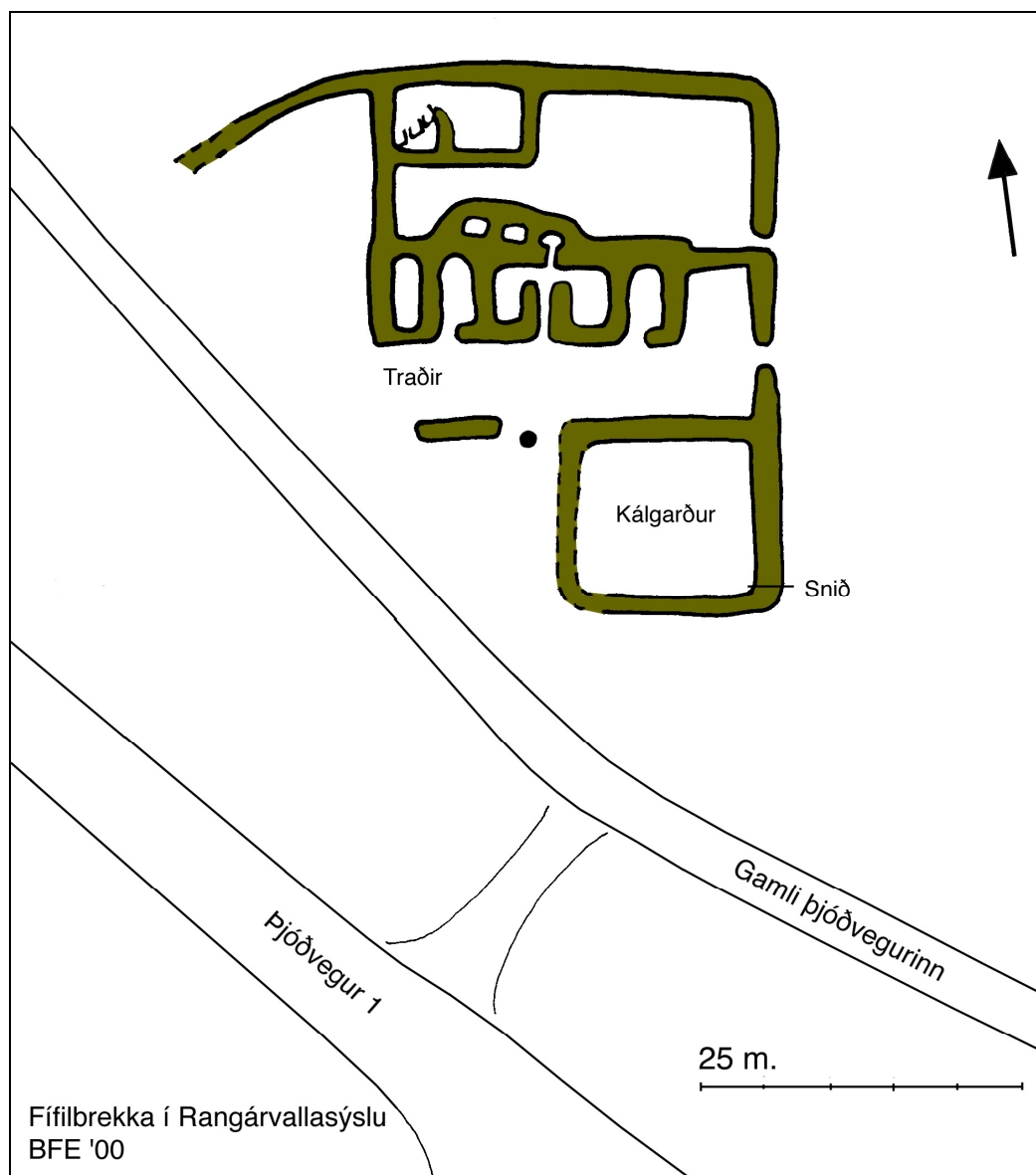
Mynd 3. Yfirlitsteikning yfir bæjarstæði Fífilbrekku. Nánari skýringar á einstökum rústum koma síðar.
