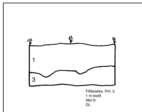
Mynd 12. Snið í prh. 5.
