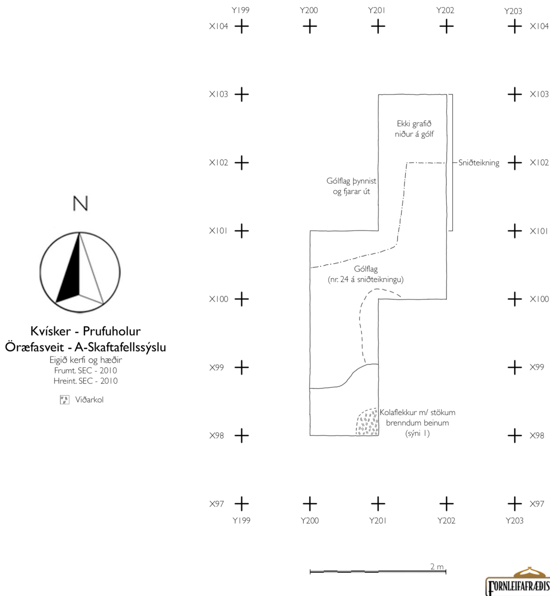
Mynd 5. Flatarteikning af prufuholunni. Aðeins er dregin upp ein mynd af hugsanlegum hólfum, eða veggjum í prufuholunni.
