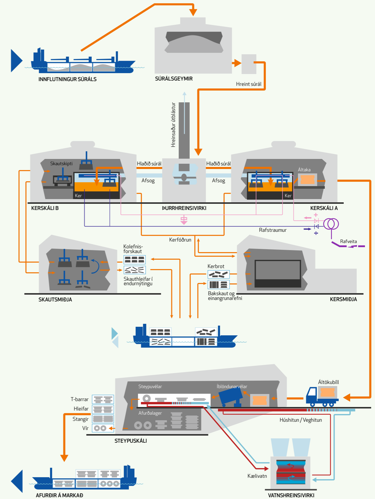
MYND 1 Framleiðsluferli í álveri Alcoa Fjarðaáls
