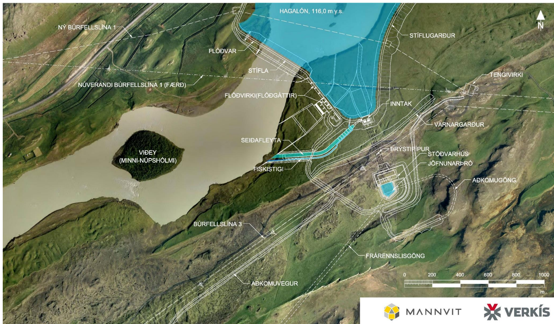
MYND 2.9 Framkvæmdasvæði Hvammsvirkjunar.
