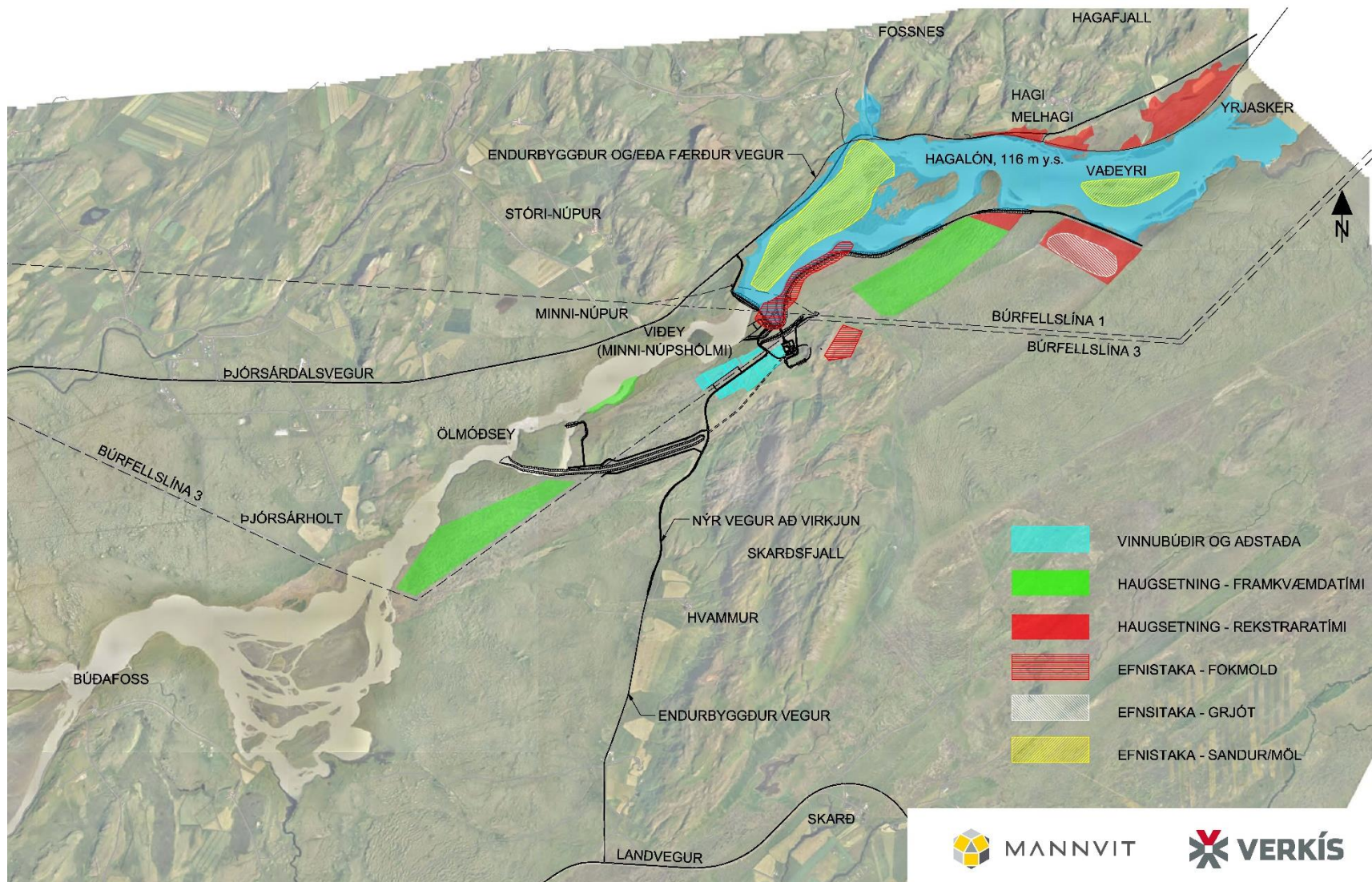
MYND 2.10 Yfirlitsmynd af fyrirhuguðum efnistöku- og haugsetningarsvæðum við fyrirhugaða Hvammsvirkjun, ásamt vinnubúðum.
