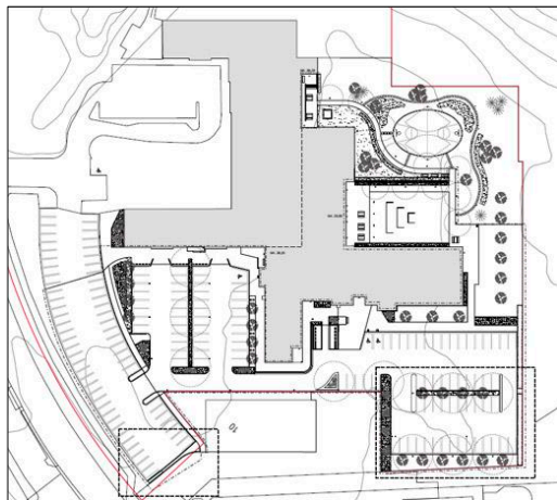
FÁ, yfirlitstekning lóðarfrágangs.
