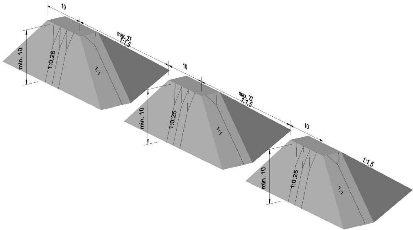
ÁSÝND Á KEILUR, HELSTU KENNISTÆRÐIR
