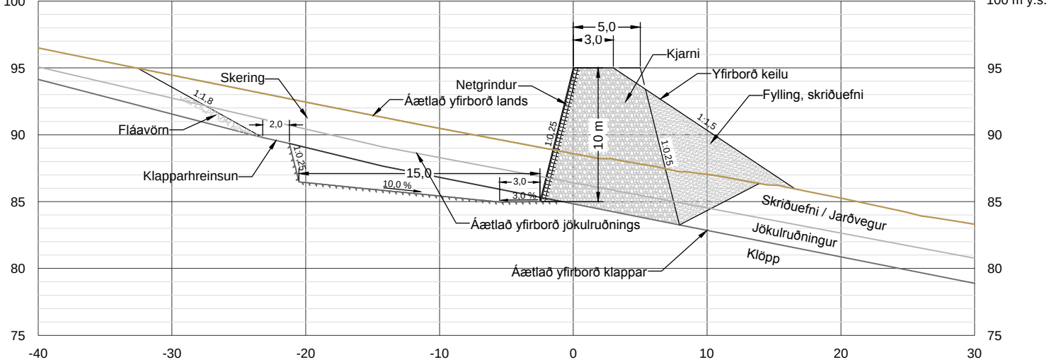
KENNISNIÐ: KEILUR Í NESGILI
