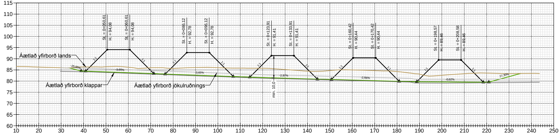
LANGSNIÐ: EFRI KEILURÖÐ, NESGILI
