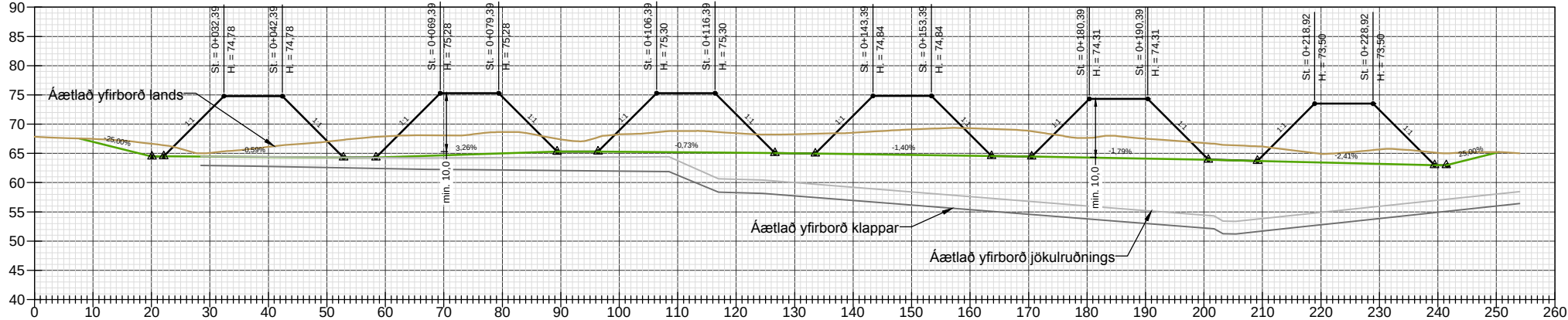
LANGSNIÐ: NEÐRI KEILURÖÐ, NESGILI
