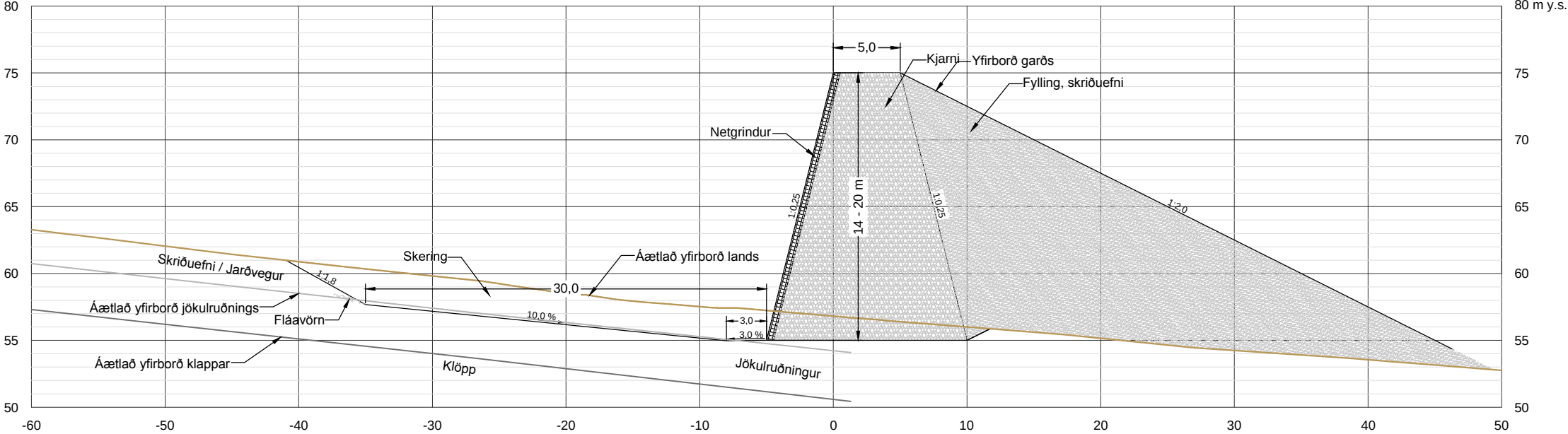
KENNISNIÐ B: ÞVERGARÐUR Í NESGILI OG BAKKAGILI
